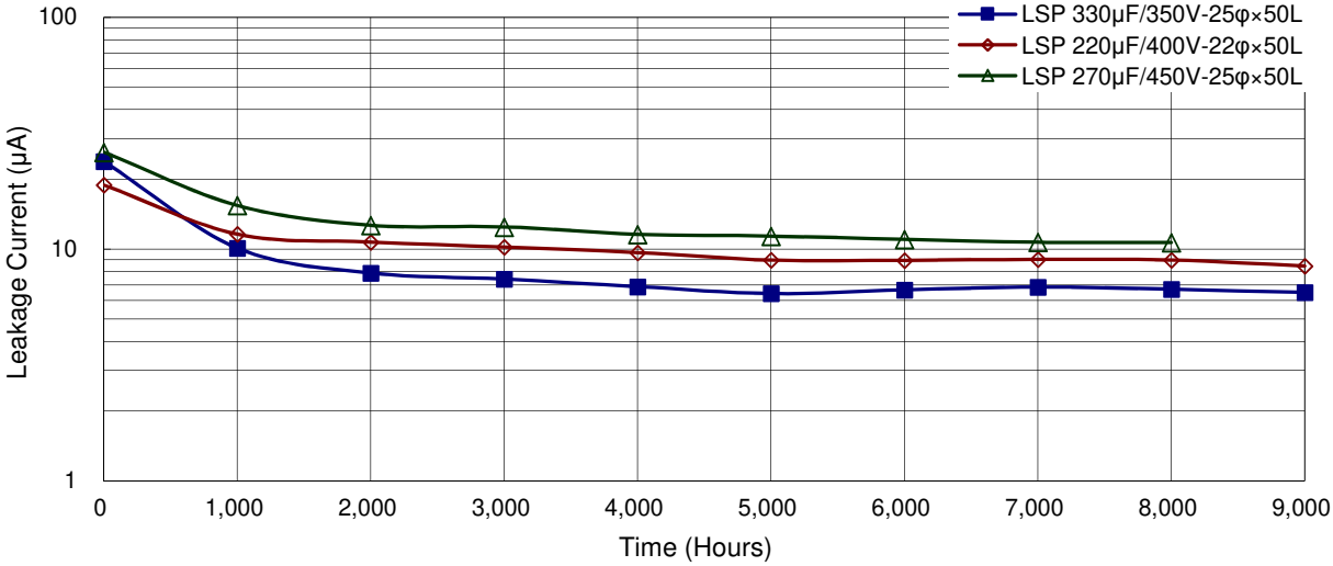
使用寿命图
