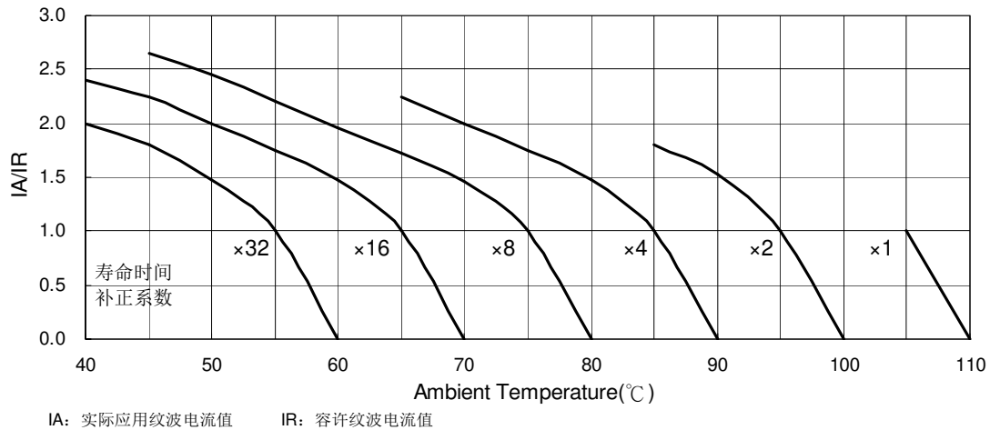
使用寿命图
