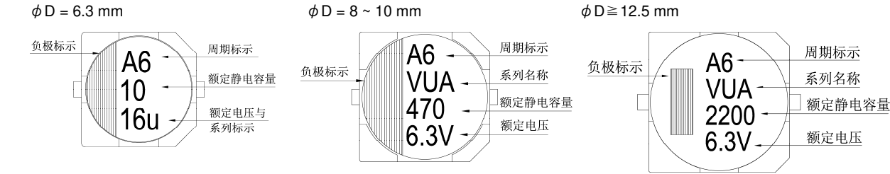
制品尺寸与容许纹波电流一览表
