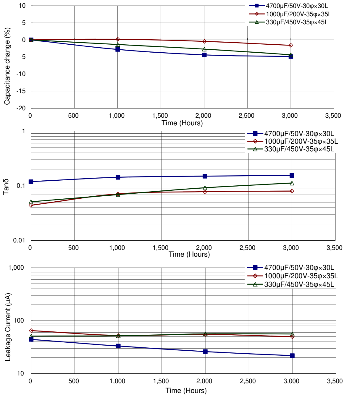
使用寿命图
