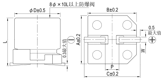
寸法图
