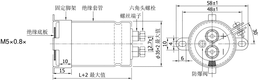
寸法图
