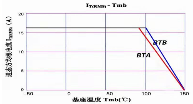
2、壳温与通态方均根电流曲线
