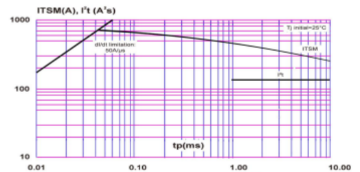
6、 I_{TSM}-t, I^2t-t 曲线
