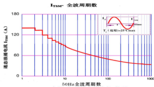
5、浪涌电流与周波数曲线
