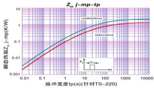
3、瞬态热阻曲线
