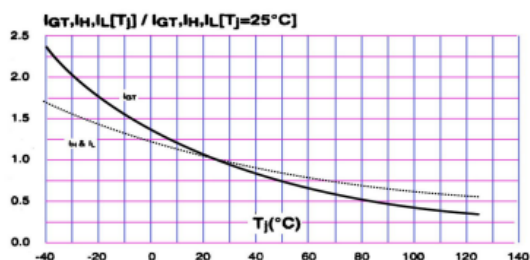
7、门极触发特性曲线
