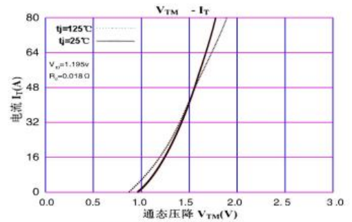
4、通态伏安特性曲线
