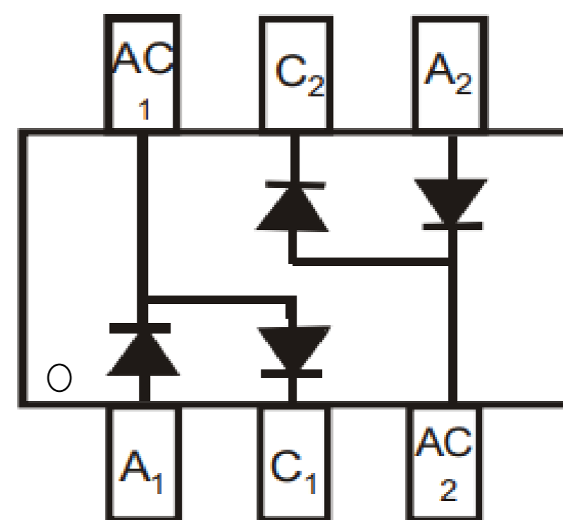
BAS70DW-04
