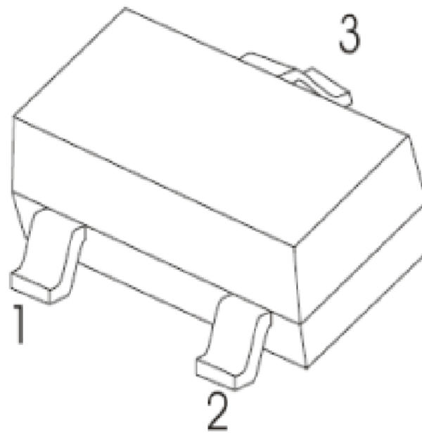
SOT-323
