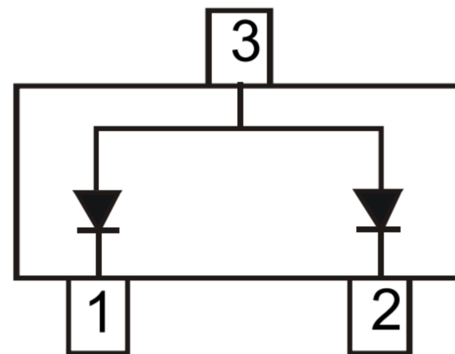
BAS70W-06
