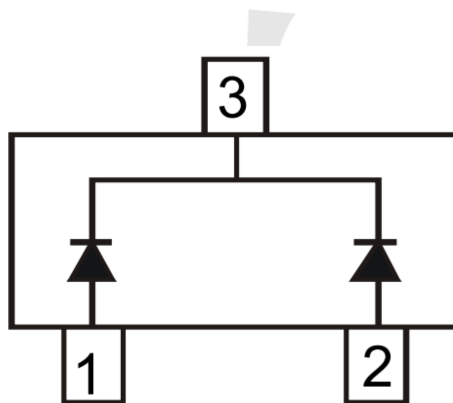
BAS40W-05
