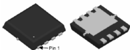
PDFN3X3-8
