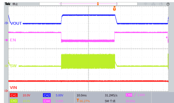
图 35.EN 引脚开关机波形 ( V_{IN}=12V , V_{OUT}=5.0V , I_{OUT}=0.5A )
