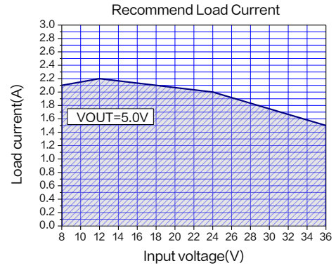
图 19.最大输出电流 ( V_{OUT}=5.0V , T_A=25^{\circ}C )
