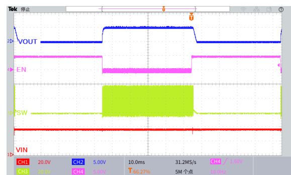
图 37.EN 引脚开关机波形 ( V_{IN}=36V , V_{OUT}=5.0V , I_{OUT}=0.5A )
