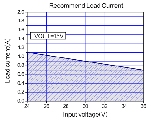
图 21.最大输出电流 ( V_{OUT}=15V , T_A=25^{\circ}C )
