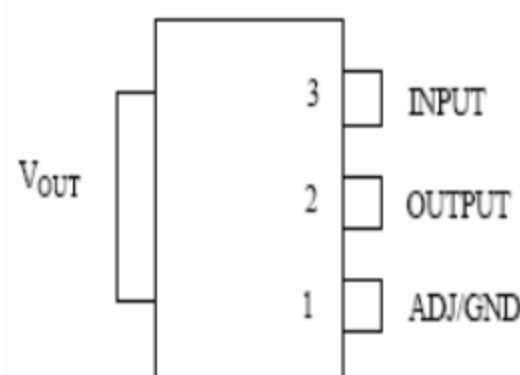
SOT-223
