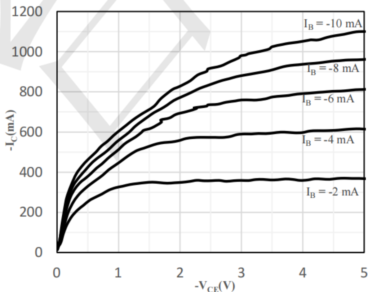
Fig 5 I_C vs. V_{CE}
