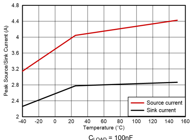
图 5-28. 峰值拉电流和灌电流
