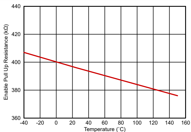
图 5-13. 使能上拉电阻
