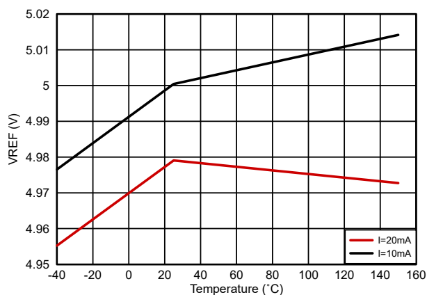
图 5-24. Vref 电压与温度间的关系
