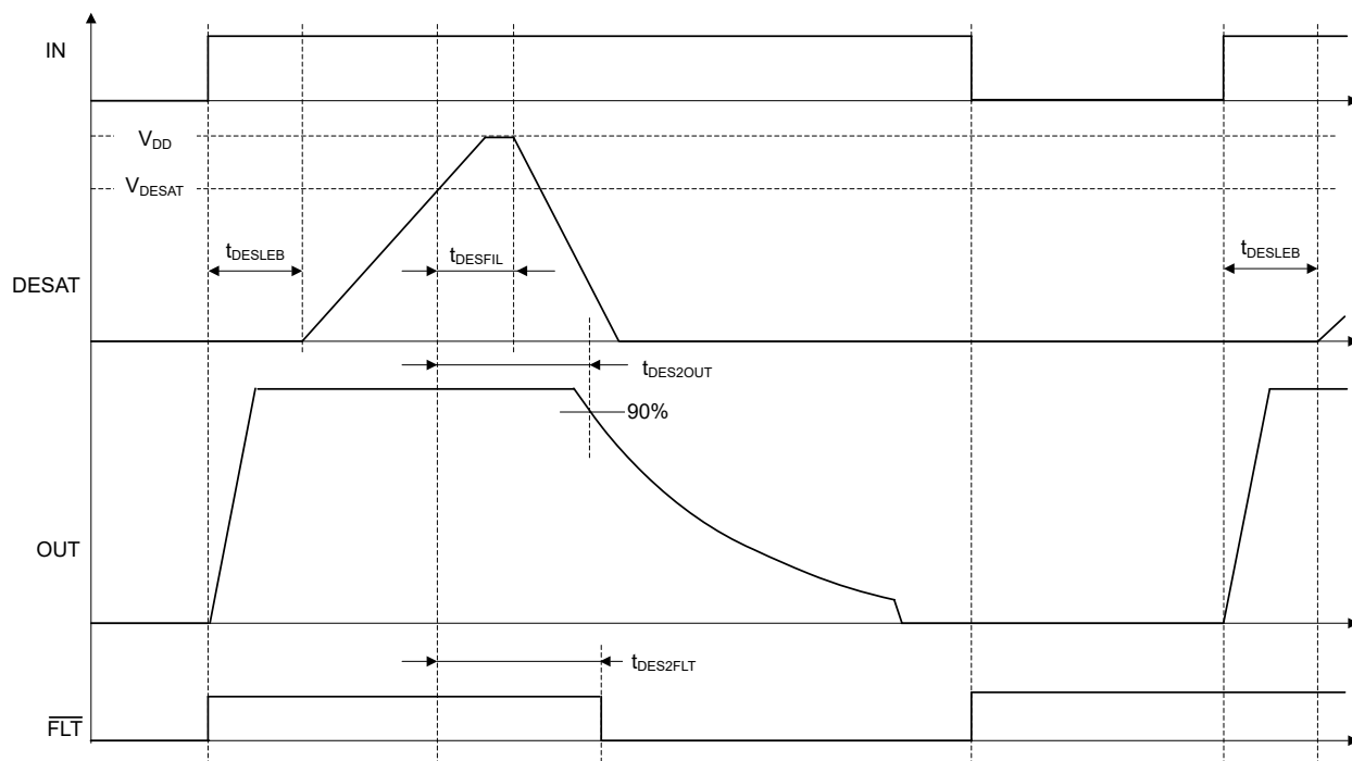
图 5-3. DESAT 保护时序图
