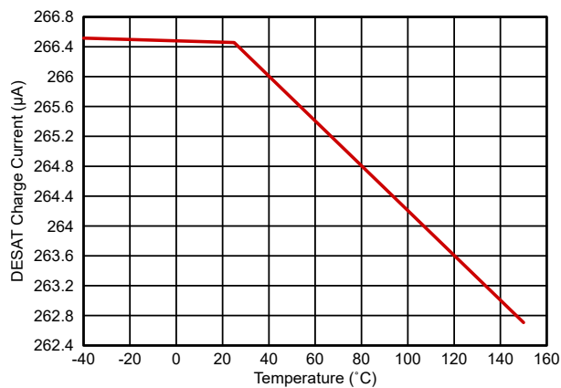
图 5-26. DESAT 充电电流与温度间的关系
