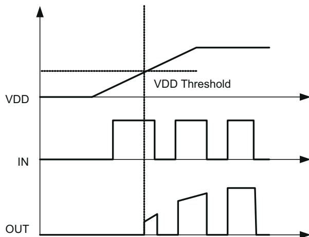
图 7-2. 上电
