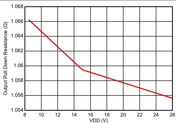
图 5-15. 输出下拉电阻
