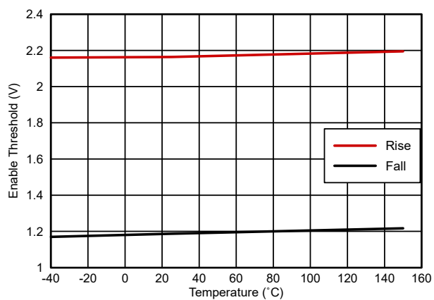
图 5-12. 使能阈值
