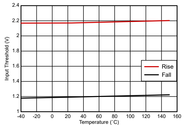
图 5-10. 输入阈值
