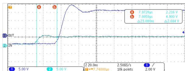
图 7-3. UCC57108 上升 (导通) 传播延迟
