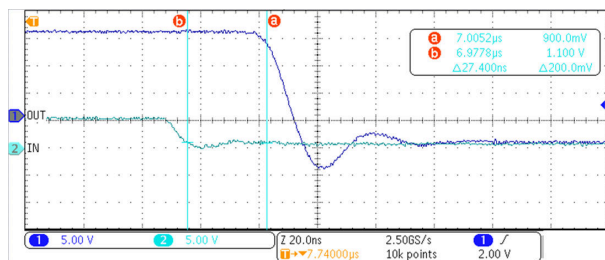
图 7-4. UCC57108-Q1 下降 ( 关断 ) 传播延迟
