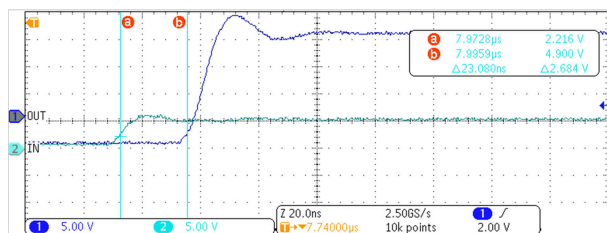
图 7-3. UCC57108-Q1 上升 ( 导通 ) 传播延迟
