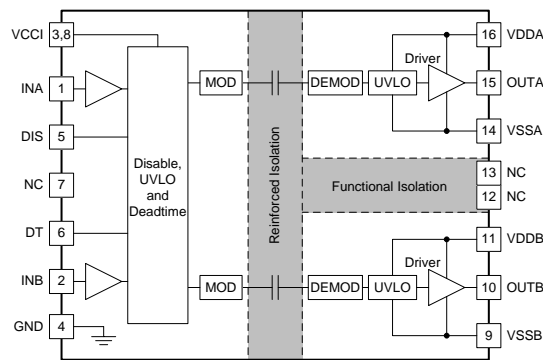
功能方框图
