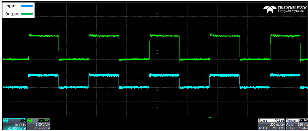
图 8-2. 上行转换 ( 1.8V 至 3.3V ) C_{LOAD} = 15pF ( 2.5MHz 时 )
