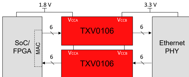
RGMII 应用中的 TXV0106
