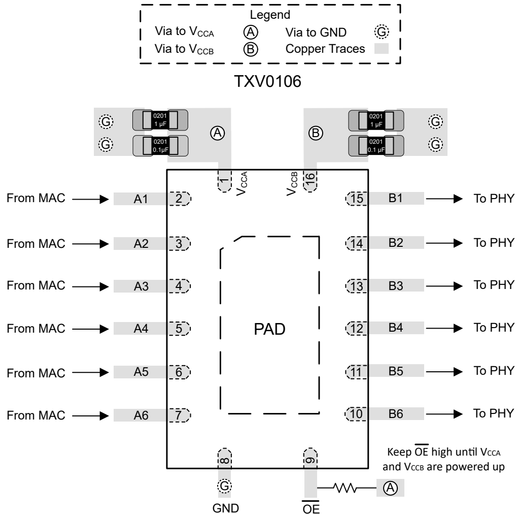
图 8-6. 布局示例 - TXV0106
