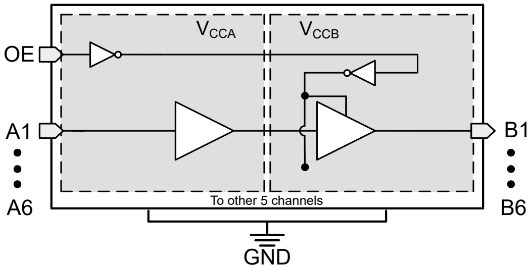
图 7-1. TXV0106 的功能方框图
