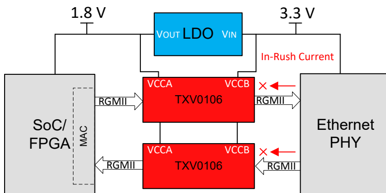
图 8-5. 使用 TXV0106 进行电源隔离
