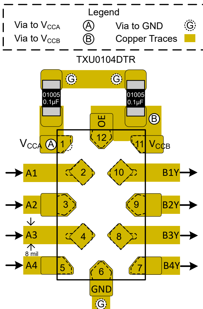
图 8-3. 布局示例 - TXU0104
