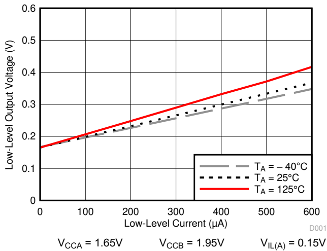
图 5-3. 低电平输出电压 ( V_{OL(Bx)} ) 与低电平电流 ( I_{OL(Bx)} ) 间的关系
