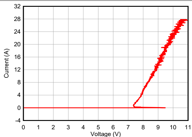
图 5-2. 负 TLP 曲线 - TSD05C
