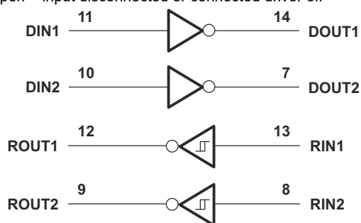
图 7-1. Logic Diagram
