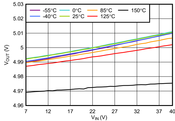
图 5-1. V_{OUT} 与 V_{IN} 间的关系 V_{OUT} = 5.0\text{V} , I_{OUT} = 10\text{mA}
