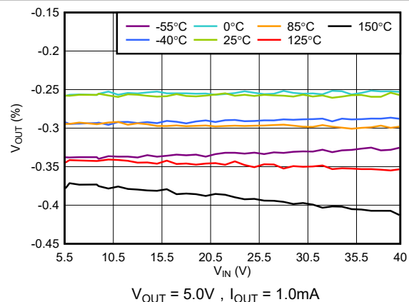
图 5-8. V_{OUT} 精度与 V_{IN} 间的关系
