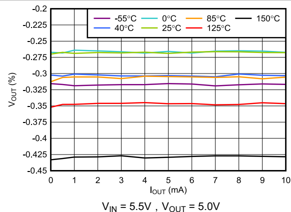
图 5-9. V_{OUT} 精度与 I_{OUT} 间的关系
