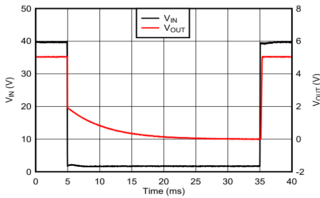
图 7-17. 欠压瞬态 (40V 至 1.7V)
