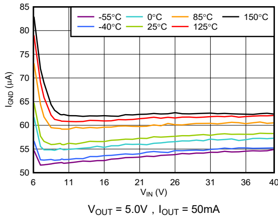
图 5-15. I_{GND} 与 V_{IN} 间的关系
