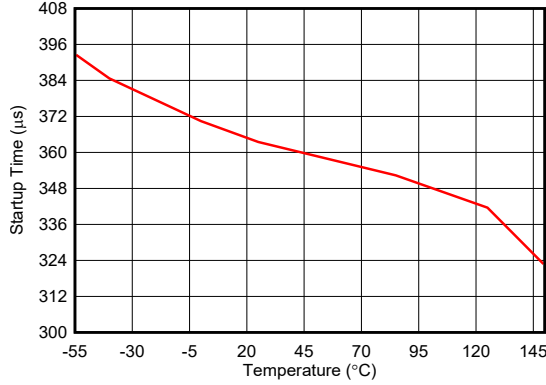
图 5-25. 软启动时间与温度间的关系
