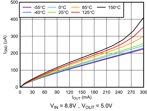
图 5-13. I_{GND} 与 I_{OUT} 间的关系
