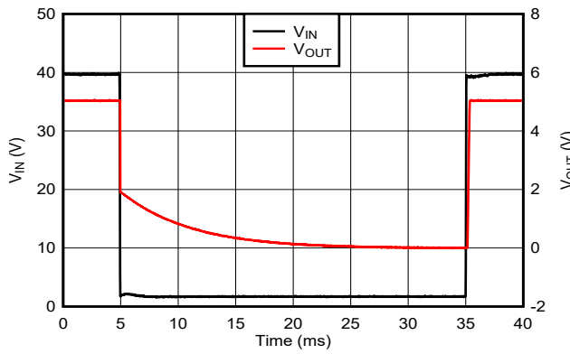
图 5-37. 欠压瞬态 (40V 至 1.7V)
