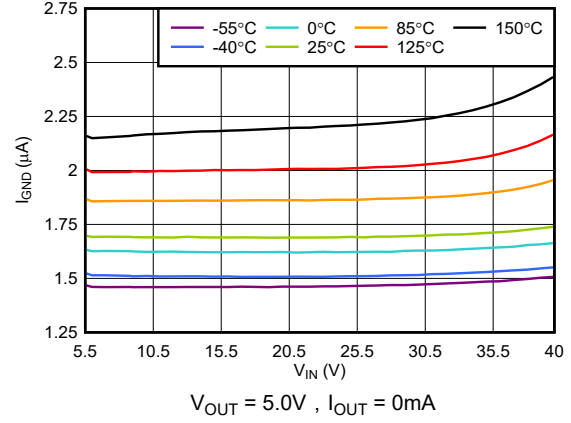
图 5-14. I_{GND} 与 V_{IN} 间的关系
