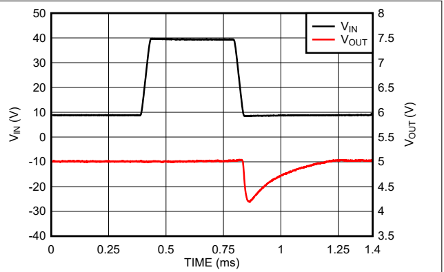
图 7-12. V_{IN} 线路瞬态 (8.8V 至 40V)
