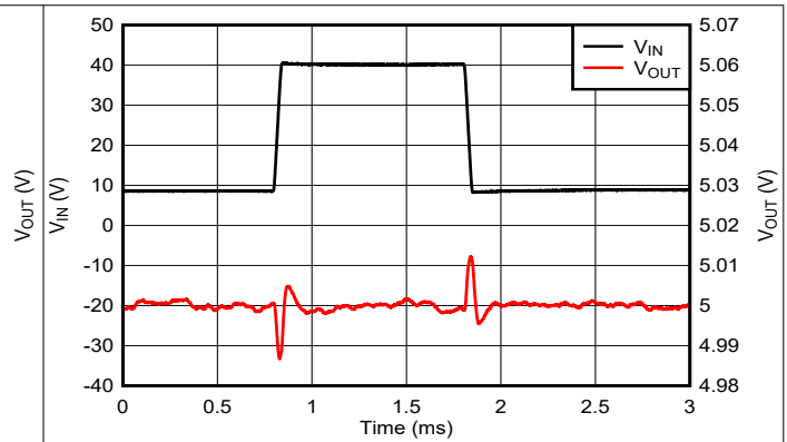
图 5-32. V_{IN} 线路瞬态 (8.8V 至 40V)
