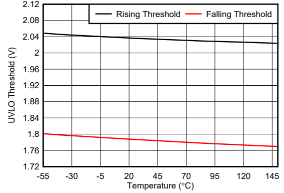
图 5-26. UVLO 阈值与温度间的关系
