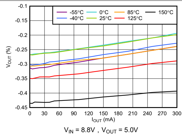
图 5-11. V_{OUT} 精度与 I_{OUT} 间的关系
