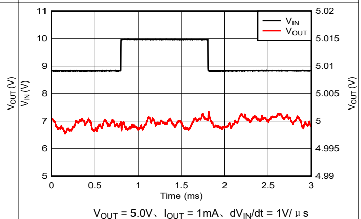
图 5-30. V_{IN} 线路瞬态 (8.8V 至 10V)
