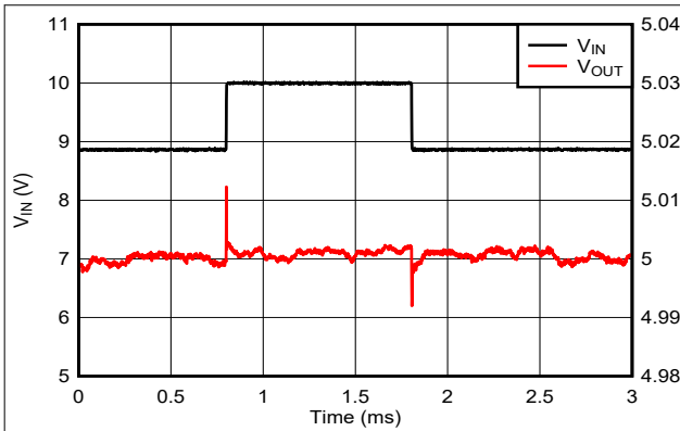
图 5-31. V_{IN} 线路瞬态 (8.8V 至 10V)
