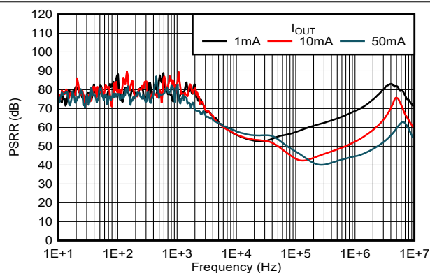
图 5-43. PSRR 与负载电流间的关系
