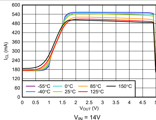
图 5-22. 电流限值与 V_{OUT} 间的关系
