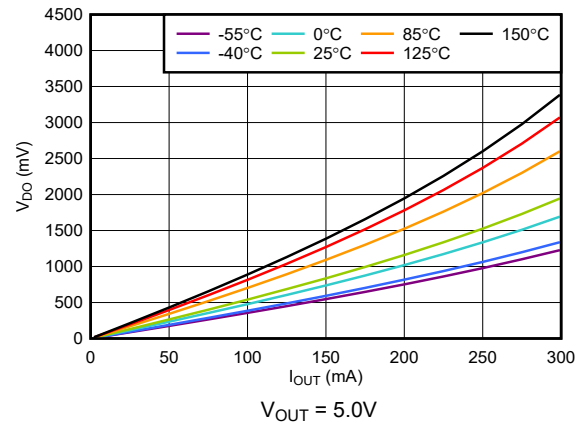
图 5-18. 压降与 I_{OUT} 间的关系
