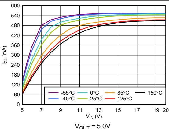
图 5-23. 电流限值与 V_{IN} 间的关系
