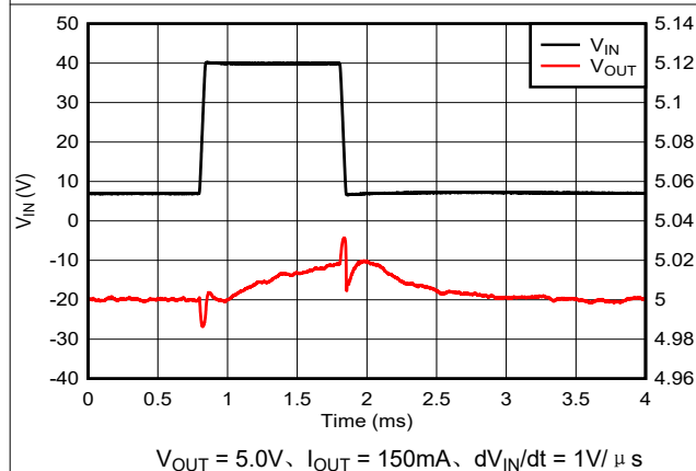
图 5-29. V_{IN} 线路瞬态 (7V 至 40V)
