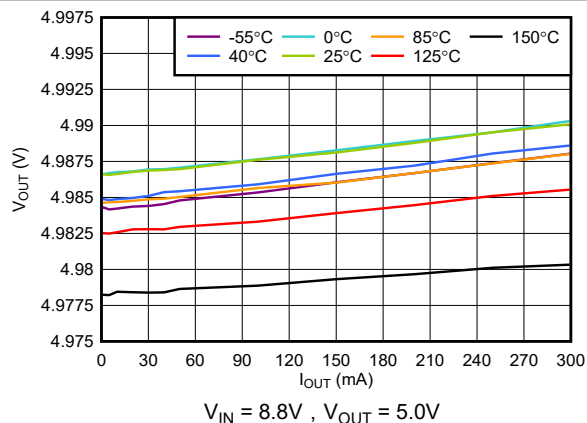
图 5-7. V_{OUT} 与 I_{OUT} 间的关系
