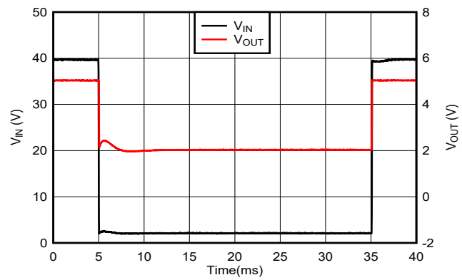
图 7-18. 欠压瞬态 (40V 至 2.1V)
