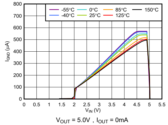
图 5-16. I_{GND} 与 V_{IN} 间的关系 (压降运行)
