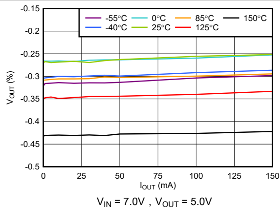
图 5-10. V_{OUT} 精度与 I_{OUT} 间的关系
