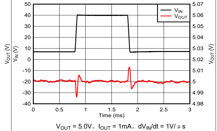
图 5-28. V_{IN} 线路瞬态 (7V 至 40V)
