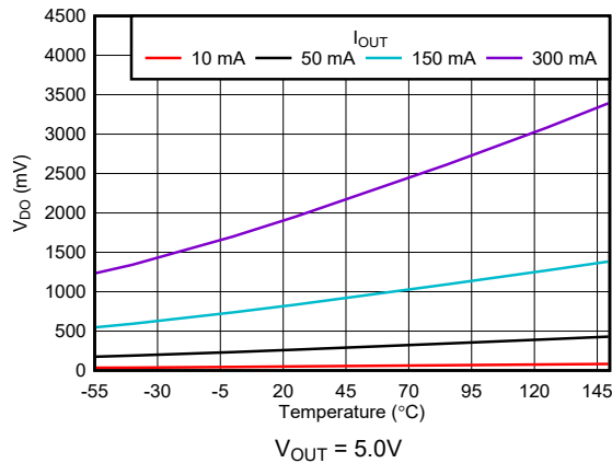
图 5-17. 压降与温度间的关系
