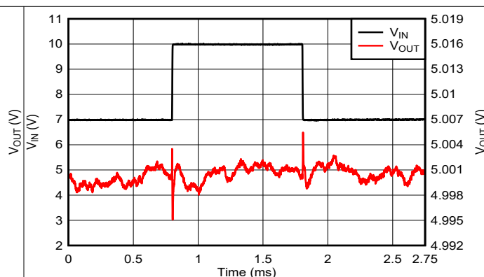
图 7-6. V_{IN} 线路瞬态 (7V 至 10V)
