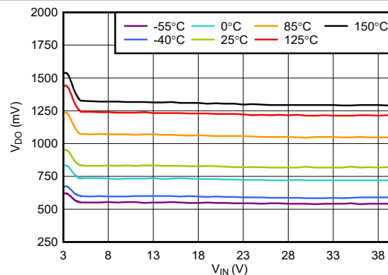
图 5-20. 压降与 V_{IN} 间的关系
