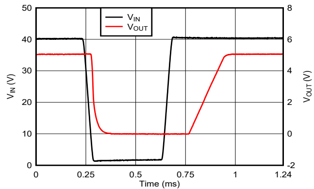
图 7-18. 欠压瞬态 (40V 至 2.1V)
