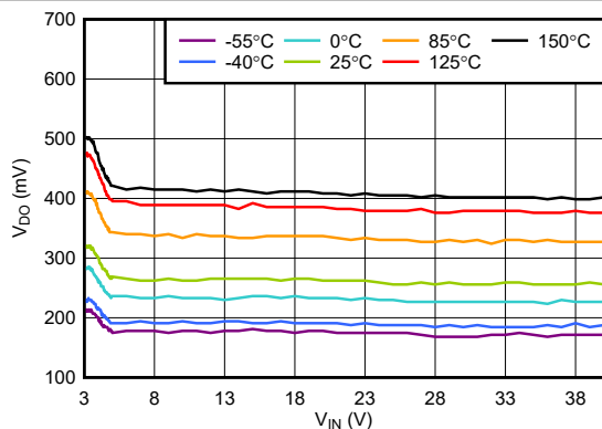
图 5-19. 压降与 V_{IN} 间的关系
