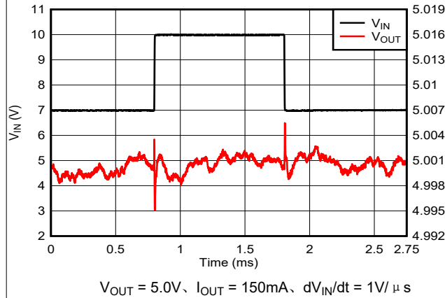
图 5-27. V_{IN} 线路瞬态 (7V 至 10V)
