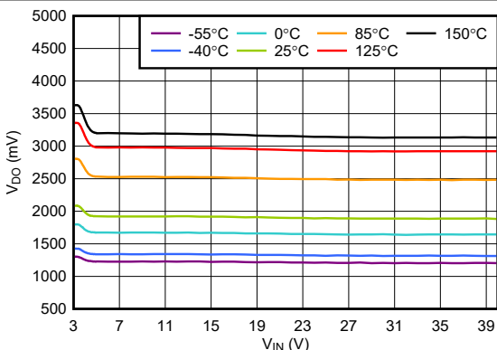
图 5-19. 压降与 V_{IN} 间的关系
