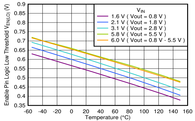
图 5-18. 使能逻辑低电平阈值与温度间的关系
