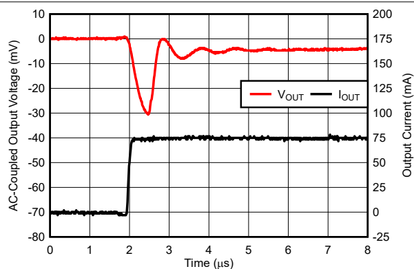
图 5-19. 负载瞬态
