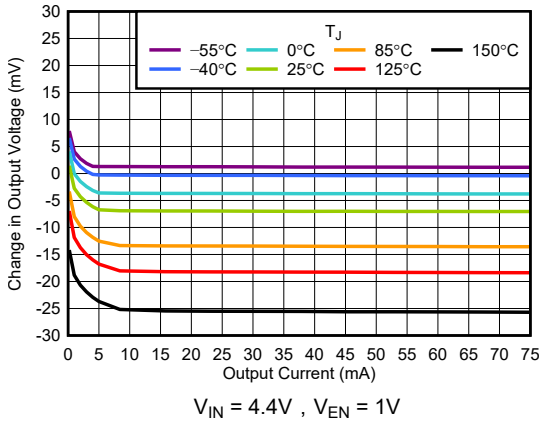
图 5-3. 负载调整率与 I_{OUT} 间的关系
