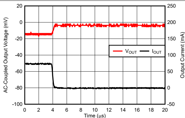
图 5-20. 负载瞬态
