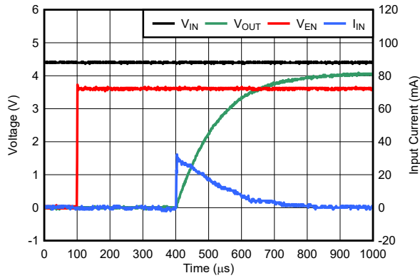
图 5-37. 启动
