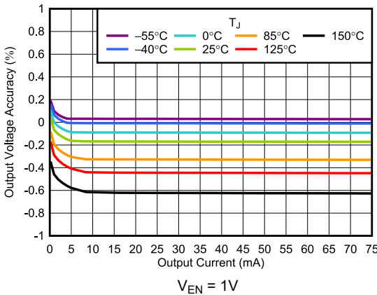
图 5-5. 输出电压精度与 I_{OUT} 间的关系
