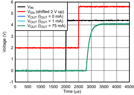
图 5-37. 启动
