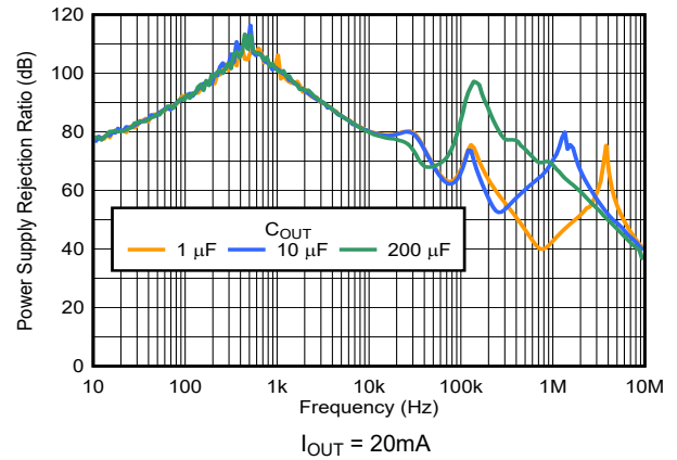
图 5-28. PSRR 与频率和 C_{OUT} 间的关系
