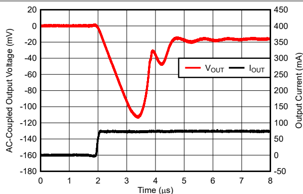
图 5-19. 负载瞬态
