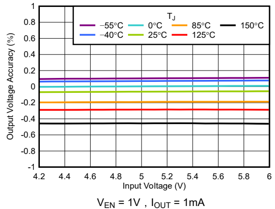
图 5-6. 输出电压精度与 V_{IN} 间的关系
