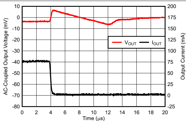
图 5-20. 负载瞬态
