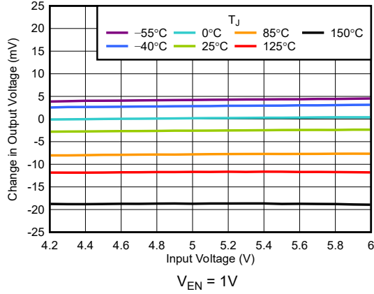
图 5-1. 线性调整率与 V_{IN} 间的关系
