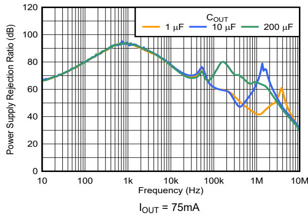
图 5-29. PSRR 与频率和 C_{OUT} 间的关系
