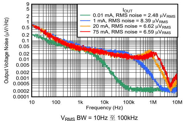
图 5-30. 噪声与频率和 I_{OUT} 间的关系
