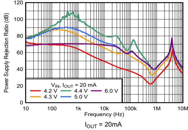
图 5-25. PSRR 与频率和 V_{IN} 间的关系
