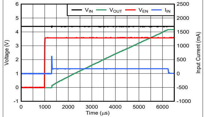
图 5-38. 启动
