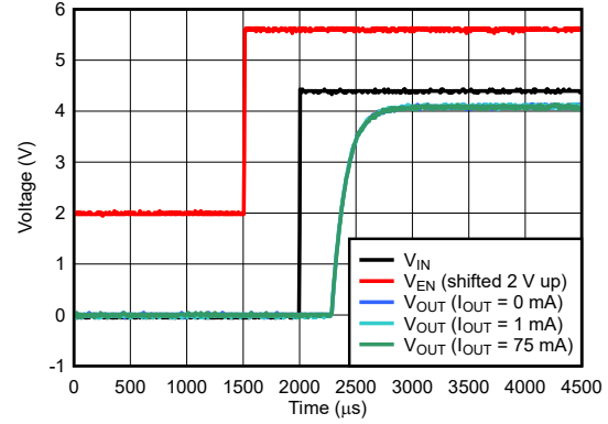
图 5-38. 启动
