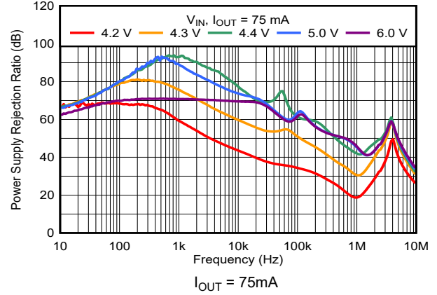
图 5-26. PSRR 与频率和 V_{IN} 间的关系
