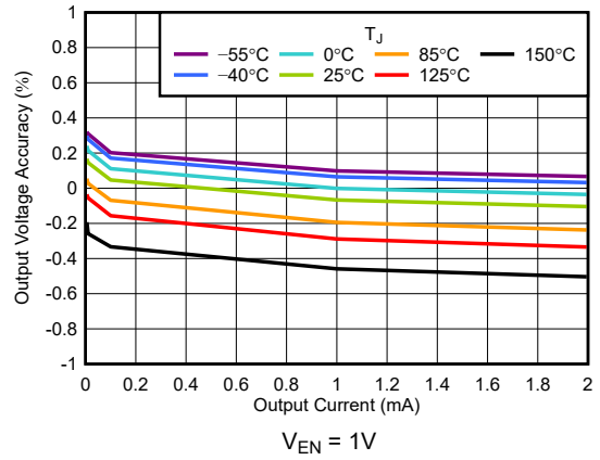
图 5-4. 输出电压精度与 I_{OUT} 间的关系
