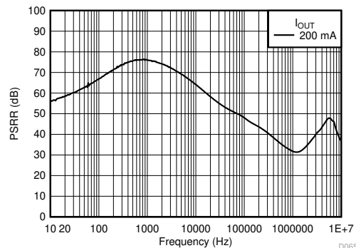
图 7-6. PSRR
