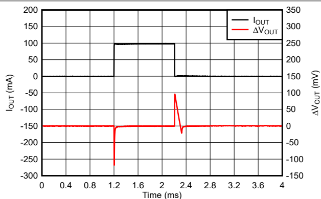
图 5-43. TPS76933-Q1 负载瞬态响应 (新芯片)
