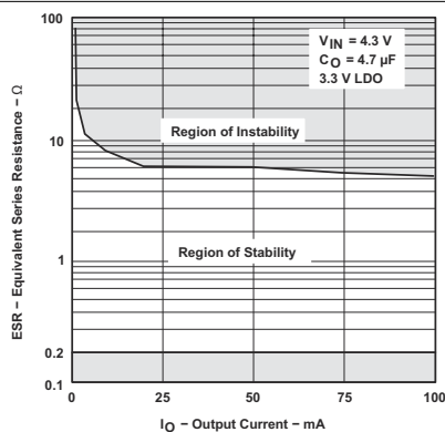
图 5-46. TPS76933-Q1 典型稳定性 ESR 区域与输出电流间的关系 (旧芯片)
