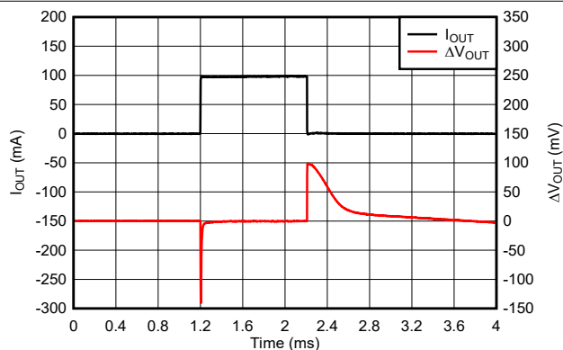
图 7-13. TPS76933-Q1 负载瞬态响应 (旧芯片)
