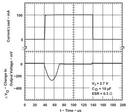
图 5-38. TPS76915-Q1 负载瞬态响应 (旧芯片)
