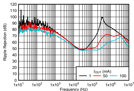
TPS76933-Q1 PSRR 与输出电流间的关系 (新芯片)
