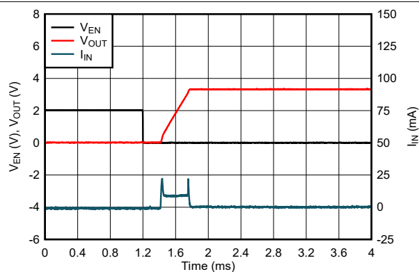
图 7-5. 断电波形 (旧芯片)
