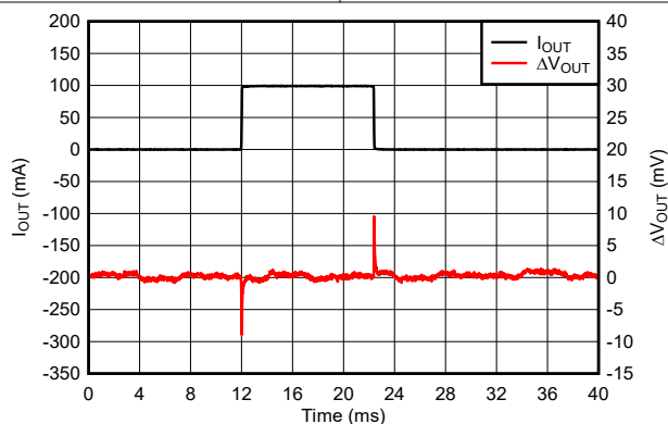
图 5-43. TPS76933-Q1 负载瞬态响应 (新芯片)
