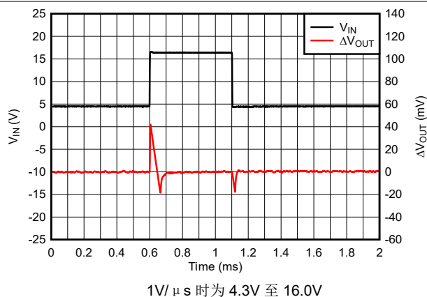
图 5-41. TPS76933-Q1 线路瞬态响应 (新芯片)
