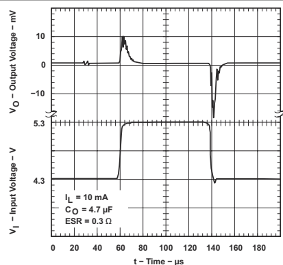
图 5-37. TPS76915-Q1 线路瞬态响应 (旧芯片)
