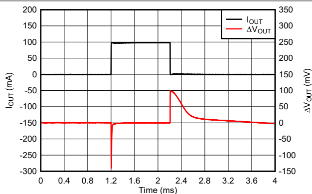
图 5-44. TPS76933-Q1 负载瞬态响应 (新芯片)
