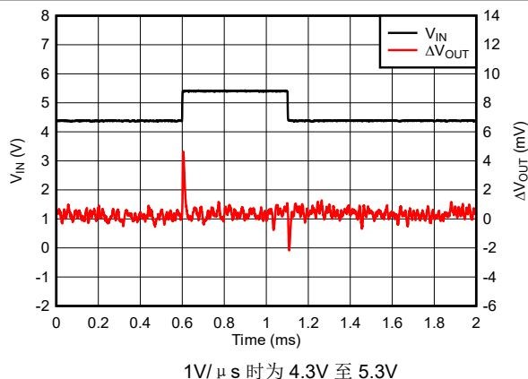
图 5-40. TPS76933-Q1 线路瞬态响应 (新芯片)
