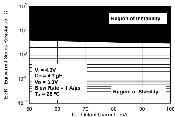
图 5-48. TPS76933-Q1 典型稳定性 ESR 区域与输出电流间的关系 (旧芯片)
