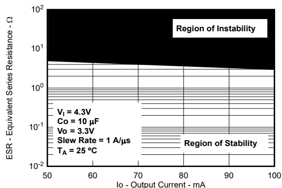
图 5-55. 典型稳定性 ESR 区域与输出电流间的关系（新芯片）
