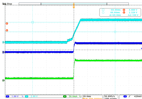
图 7-4. 上电波形 (旧芯片)
