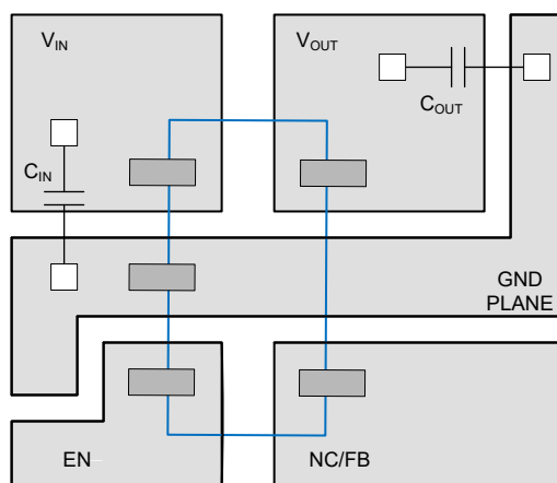
图 7-17. 布局建议
