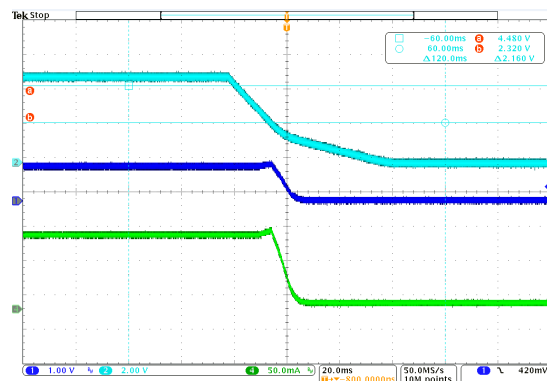
图 7-5. 断电波形 (旧芯片)
