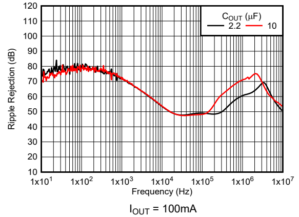
图 5-32. TPS76933-Q1 纹波抑制与输出电容器间的关系 (新芯片)
