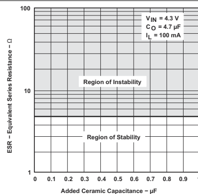
图 5-47. TPS76933-Q1 典型稳定性 ESR 区域与添加的陶瓷电容间的关系 (旧芯片)
