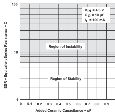
图 5-47. TPS76933-Q1 典型稳定性 ESR 区域与添加的陶瓷电容间的关系 (旧芯片)
