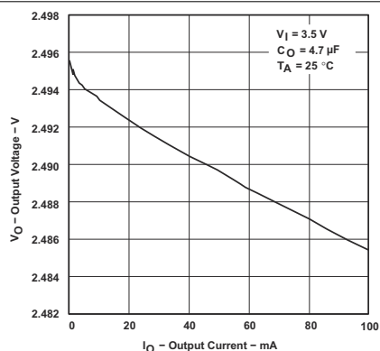
图 5-1. TPS76925-Q1 输出电压与输出电流间的关系 (旧芯片)
