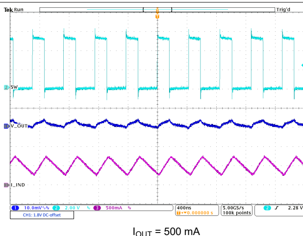
图 8-20. PWM Operation
