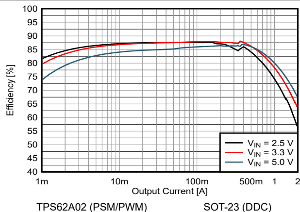
图 8-16. 0.6V Output Efficiency
