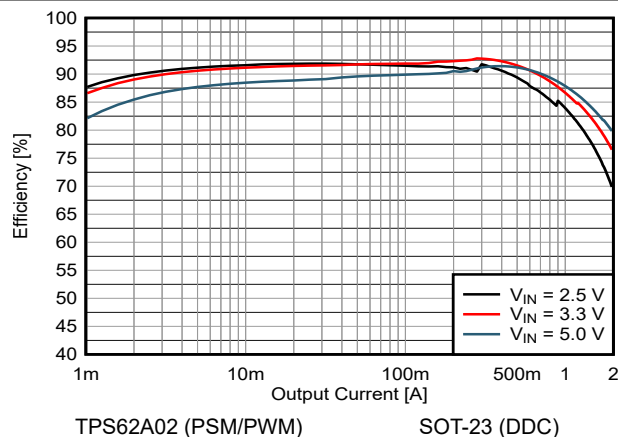
图 8-17. 1.2V Output Efficiency
