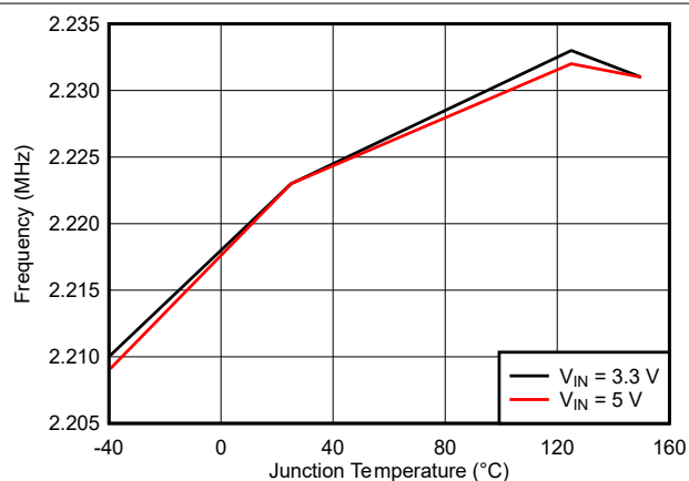
图 7-4. 开关频率与温度间的关系
