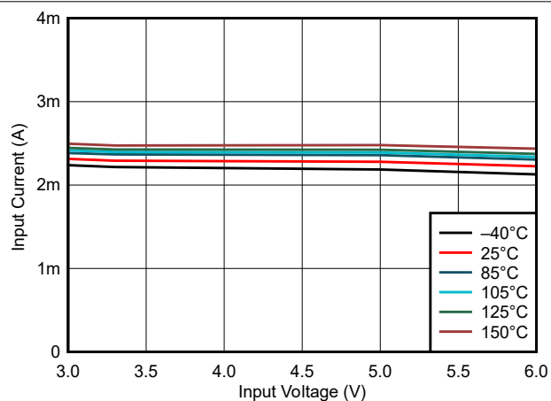
图 7-1. 工作电源电流 (节能模式)
