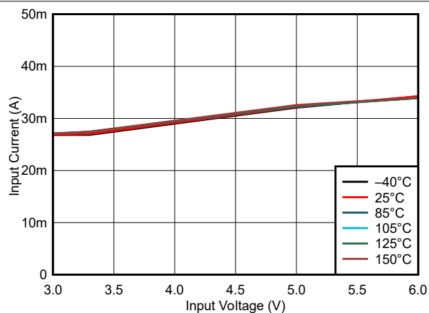
图 7-2. 工作电源电流 (强制 PWM)
