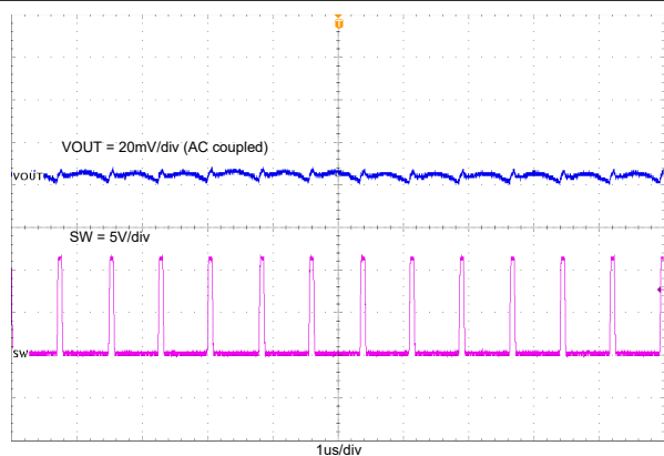
图 7-4. TPS561243 输出电压纹波 (1A 负载)
