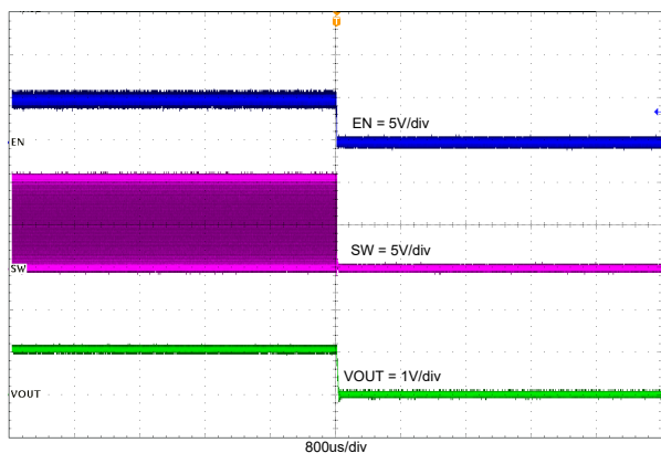
图 7-9. TPS561246 在负载电流为 1A 时使能关
