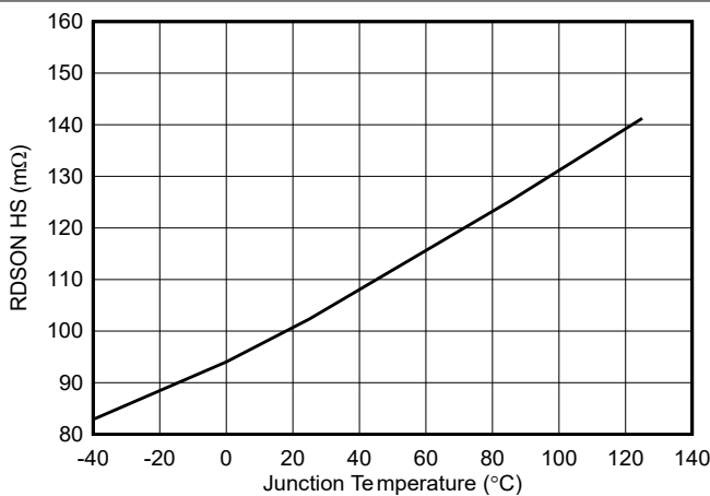
图 5-5. 低侧 Rdson
