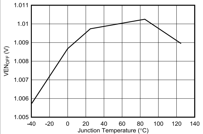
图 5-4. 使能关闭阈值电压
