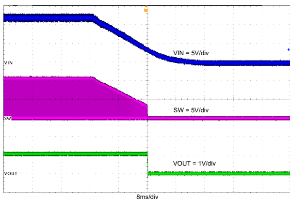
图 7-13. TPS561246 在负载电流为 1A 时断电
