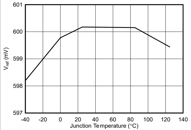
图 5-2. Vref 电压
