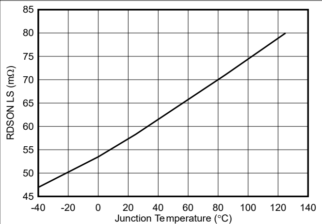
图 5-6. 高侧 Rdson
