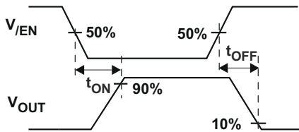
图 6-4. 使能时序，低电平有效使能
