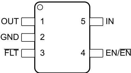
图 5-3. DBV 封装 5 引脚 SOT-23 顶视图
