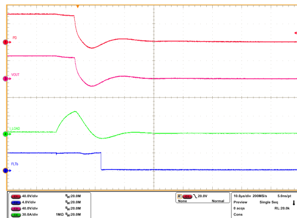
图 9-9. TPS12100-Q1 器件的输出短路响应
