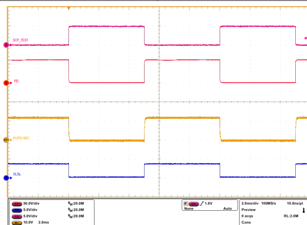
图 9-10. TPS12100-Q1 的短路保护诊断测试响应
