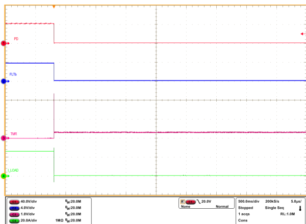
图 9-8. TPS12100-Q1 针对过流故障的闭锁响应
