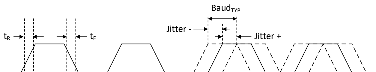
图 6-1. SMAART Wire™/UART 接口时序图
