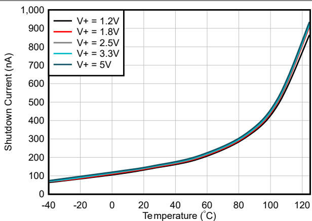
图 6-7. 关断电流与温度间的关系
