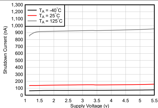
图 6-4. 关断电流与电源电压间的关系
