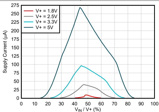
图 6-16. 电源电流与输入电池输入电压间的关系
