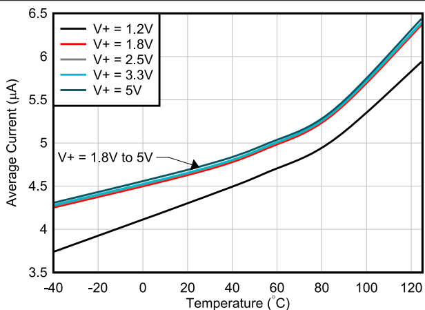
图 6-5. 平均静态电流与温度间的关系
