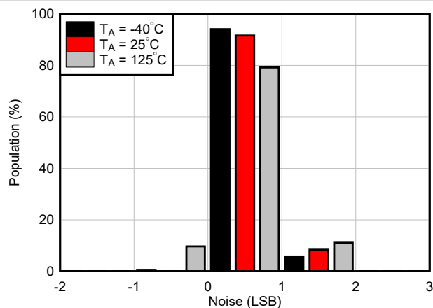
图 6-15. 噪声直方图 (油浴测量)
