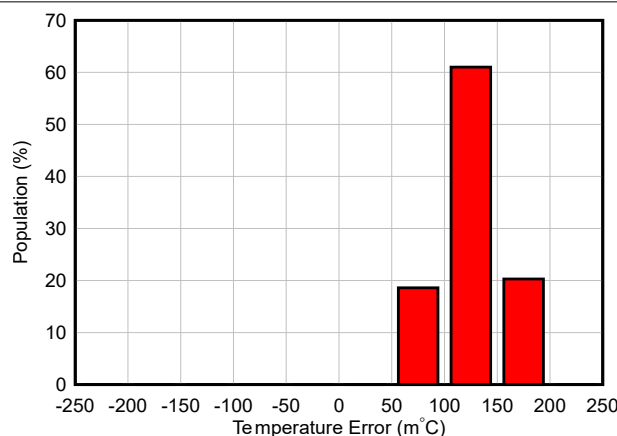
图 6-12. 25 ^\circ\text{C} 时的温度误差
