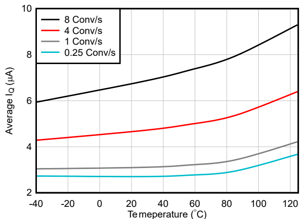
图 6-11. 平均电源电流与转换率间的关系
