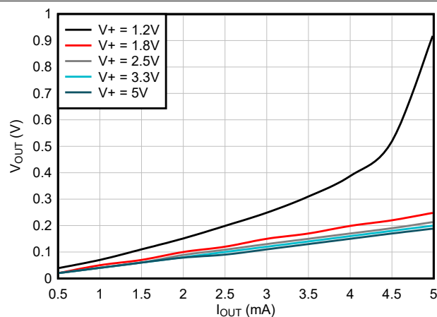
图 6-14. ALERT 引脚输出电压与引脚灌电流间的关系
