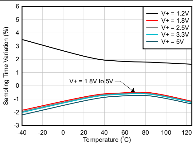
图 6-13. 采样时间与温度间的关系
