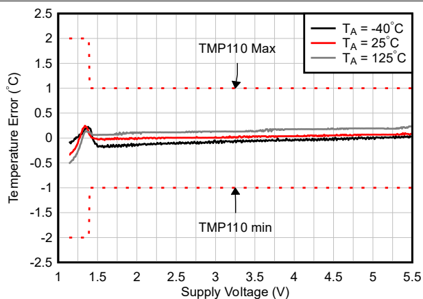
图 6-3. 温度误差与电源电压间的关系
