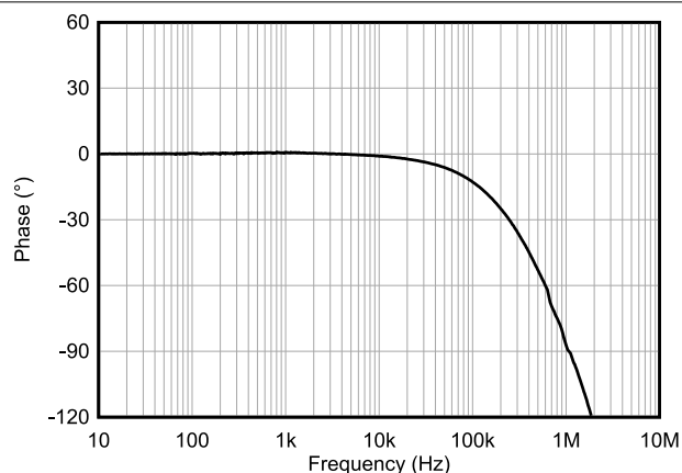
图 6-6. 相位与频率间的关系 (所有增益)
