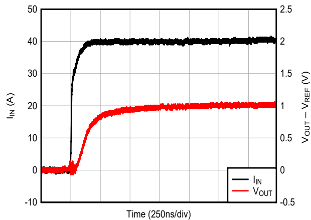
图 6-9. 电压输出阶跃响应 (上升)
