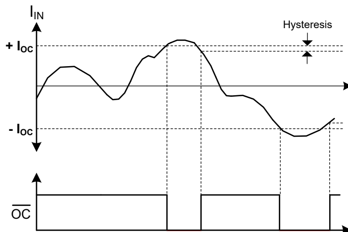
图 8-7. 过流检测图
