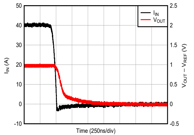
图 6-10. 电压输出阶跃响应 (下降)
