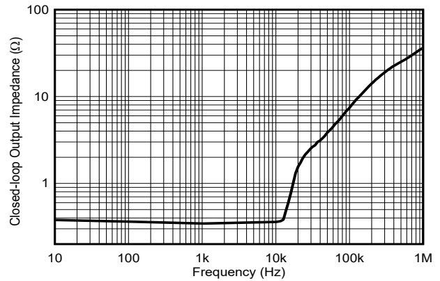
图 6-8. 输出阻抗与频率间的关系
