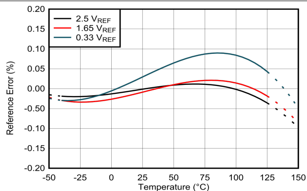
图 6-2. 基准误差与温度间的关系
