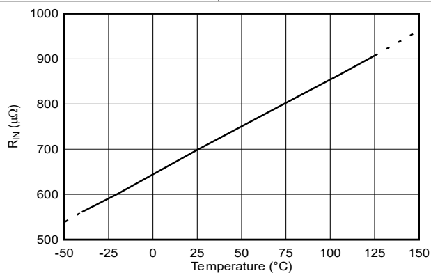
图 6-15. 输入导体电阻与温度间的关系
