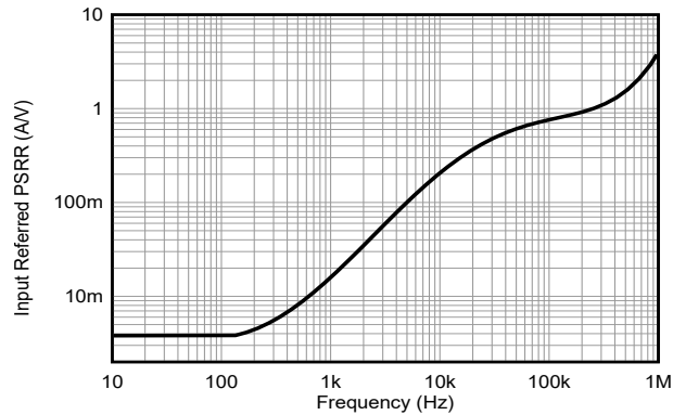
图 6-7. PSRR 与频率间的关系
