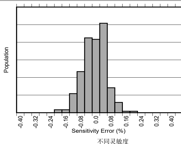
图 6-4. 灵敏度误差产生分布图：A 级
