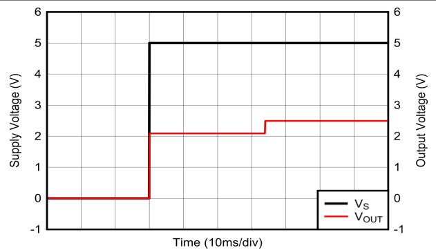
图 6-12. 启动瞬态响应
