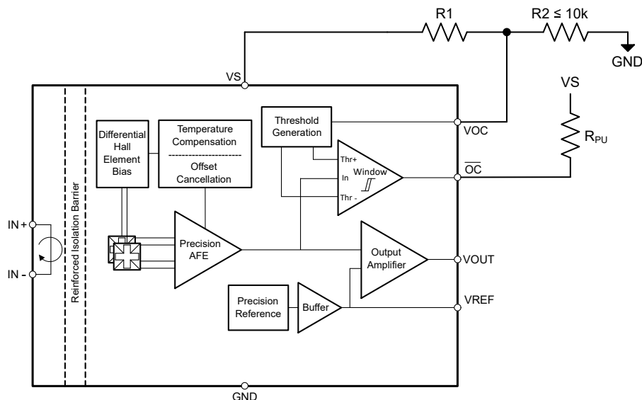
图 8-5. 使用电源电压的用户可配置过流阈值
