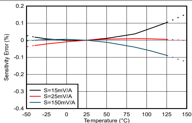
图 6-1. 灵敏度误差与温度间的关系
