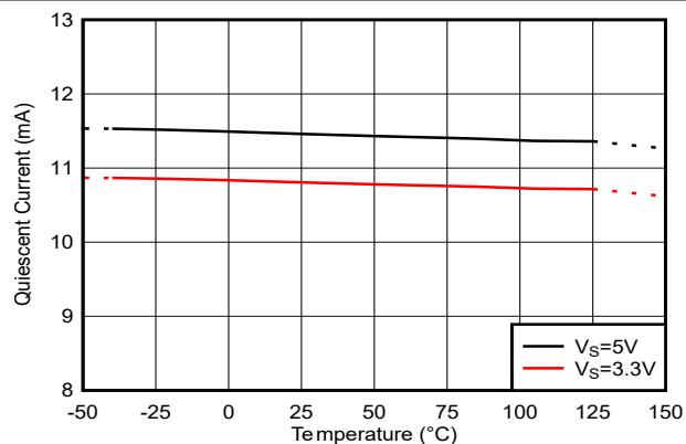
图 6-14. 静态电流与温度间的关系
