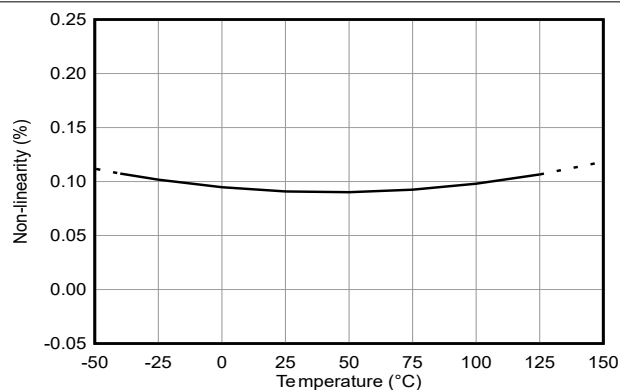
图 6-3. 非线性与温度间的关系
