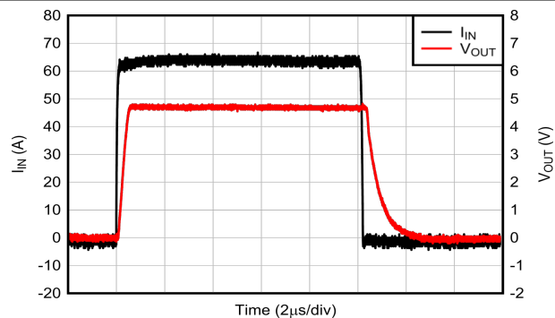
图 6-11. 电流过载响应
