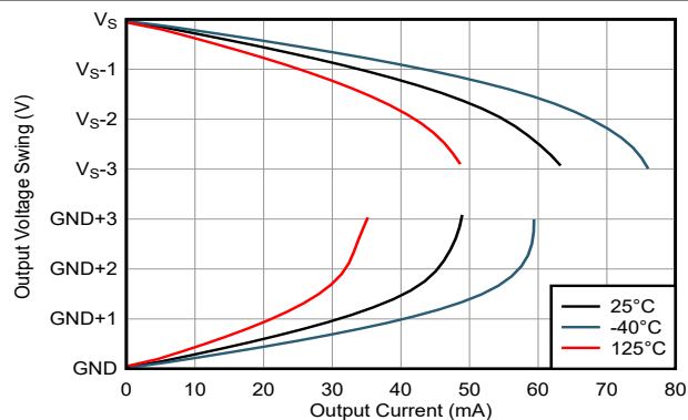
图 6-13. 输出摆幅与输出电流间的关系
