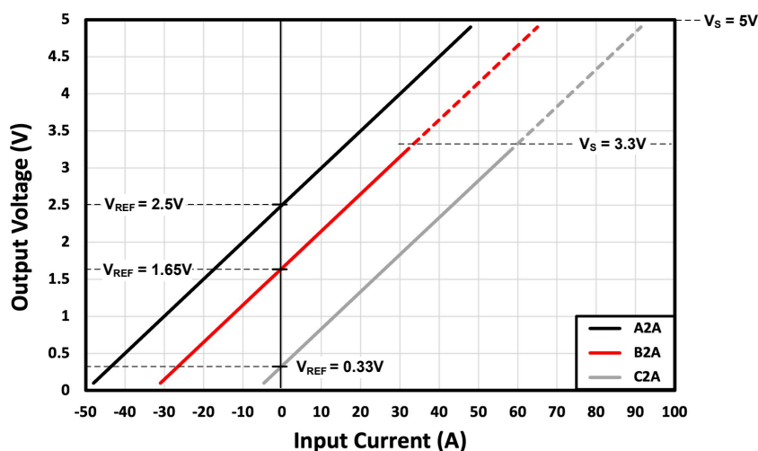
图 8-4. TMCS1126x2A 的输出电压与输入电流之间的关系
