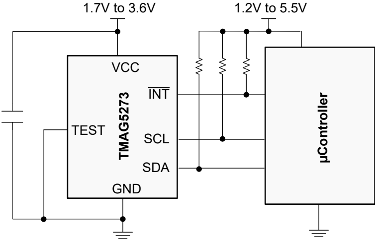
应用方框图
