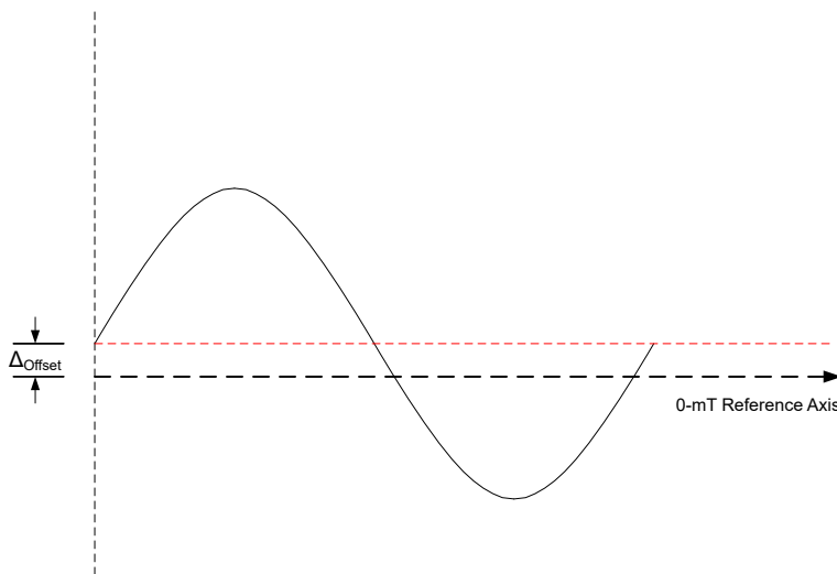
图 6-19. 磁传感器数据偏移校正
