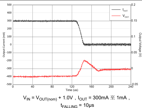
图 5-12. 负载瞬态
