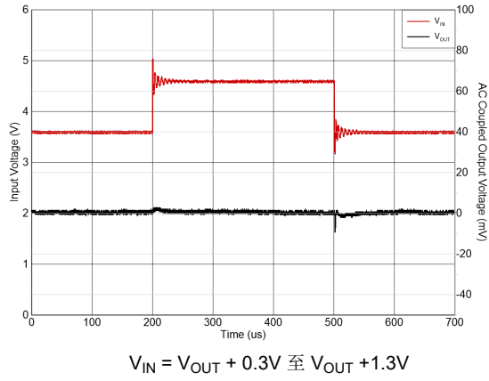
图 5-13. 线路瞬态
