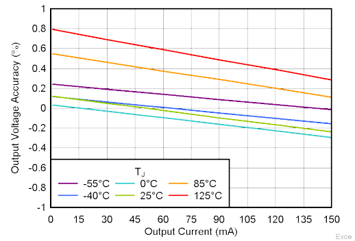
图 5-2. 负载调整率与 I_{OUT} 间的关系
