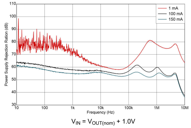
图 5-14. PSRR 与频率间的关系
