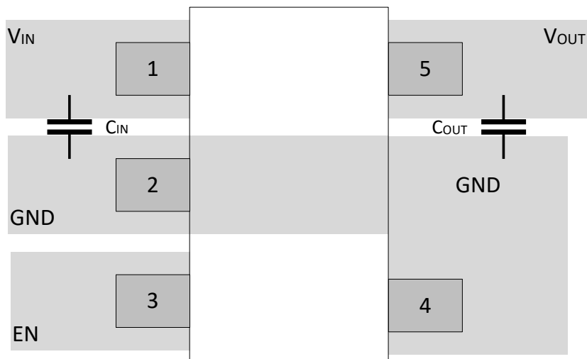
图 7-4. DBV 封装 (SOT-23) 典型布局
