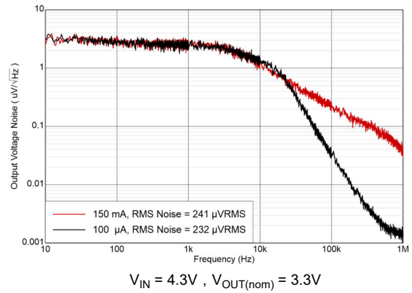
图 5-16. 噪声
