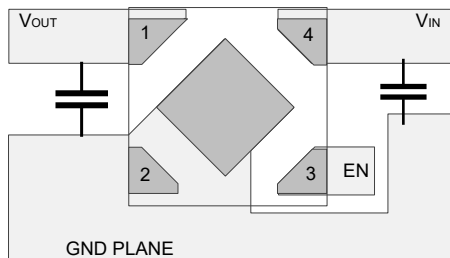
图 7-5. DQN 封装 (X2SON) 典型布局
