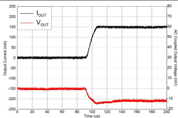
图 5-9. 电流限制
