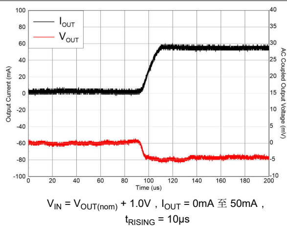
图 5-11. 负载瞬态
