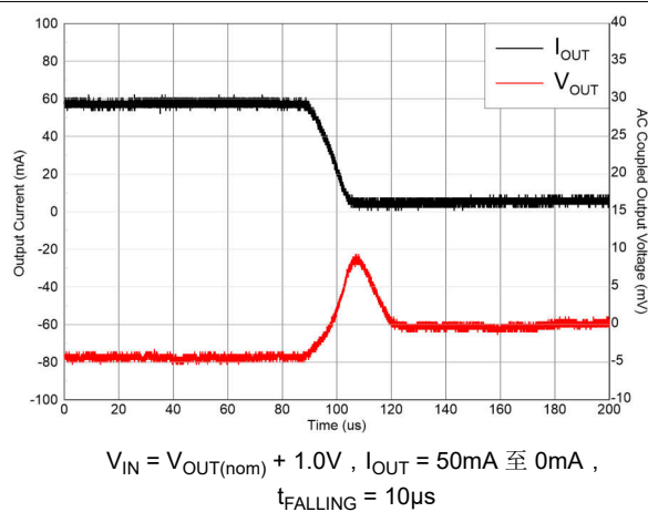
图 5-12. 负载瞬态
