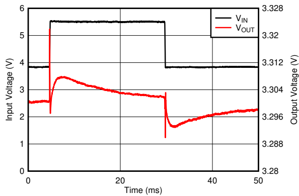
图 5-7. Line Transient
