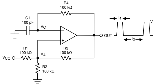
图 8-9. Square-Wave Oscillator
