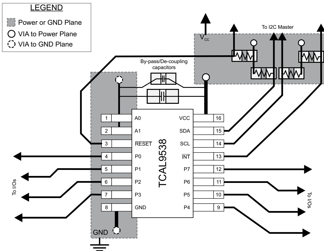
图 8-9. TCAL9538 布局
