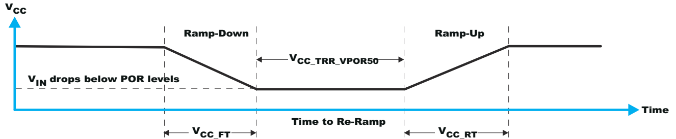
图 8-6. 将 V 降至低于 POR 阈值，然后重新上升
