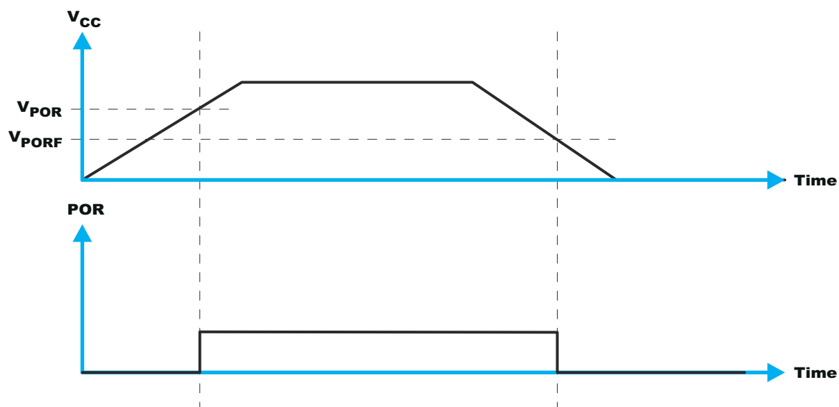
图 8-8. V_{POR}
