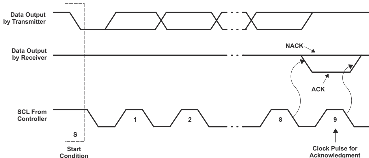
图 7-6. I 2 C 总线上的确认
