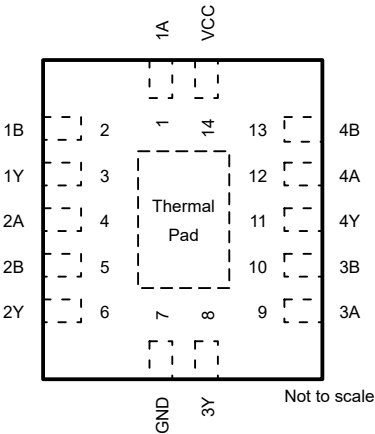
图 4-1. BQA 封装，14 引脚 WQFN (顶视图)
