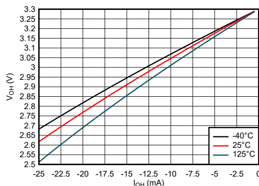
图 5-2. 高电平状态下输出电压与电流间的关系 (3.3V 电源)
