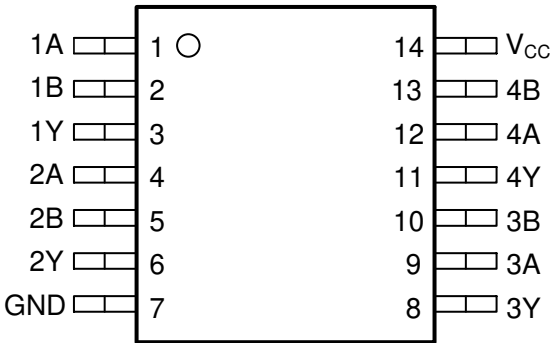
图 4-2. D 或 PW 封装，14 引脚 TSSOP (顶视图)
