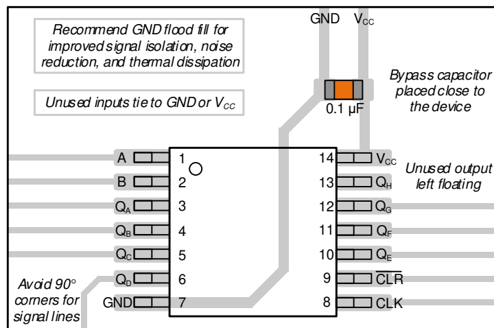
图 8-3. SN74AHC164-Q1 的示例布局
