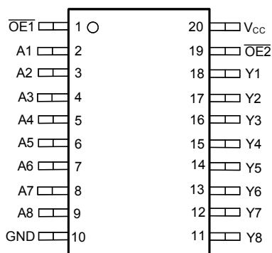
图 4-1. PW 和 DGS 封装， 20 引脚 TSSOP 和 VSSOP (顶视图)
