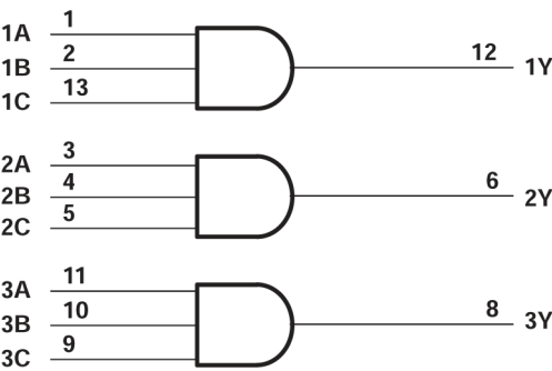
图 6-1. 逻辑图，每个逻辑门（正逻辑）
