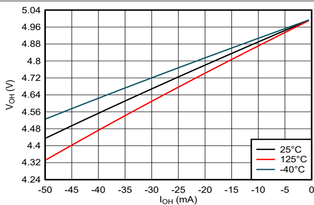
图 5-6. 高电平状态下输出电压与电流间的关系 (5V 电源)
