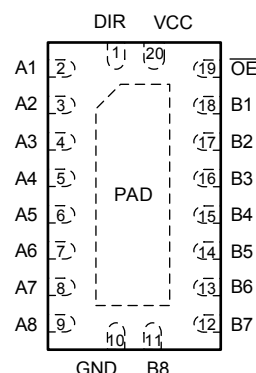
图 4-2. RKS 封装，20 引脚 VQFN (俯视图)
