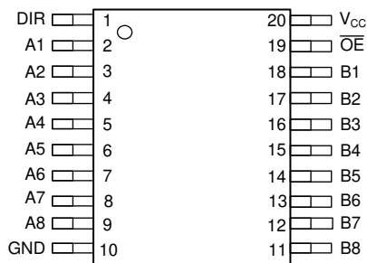
图 4-1. DGS 或 PW 封装，20 引脚 VSSOP 或 TSSOP (顶视图)
