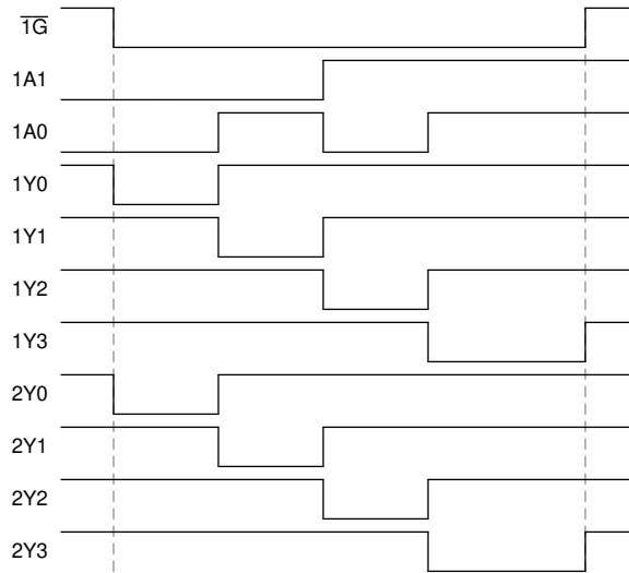
图 8-2. 应用时序图
