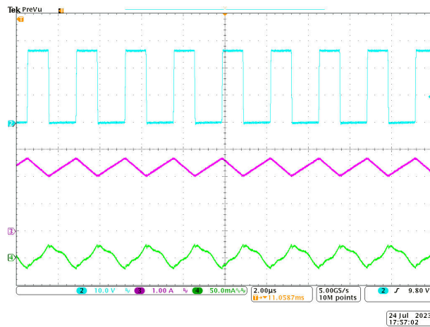
通道 2 : SW, 通道 3 : 电感器电流, 通道 4 : LED 电流纹波 (交流)
