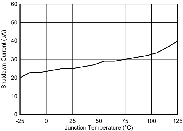
图 6-2. 关断电流与结温间的关系
