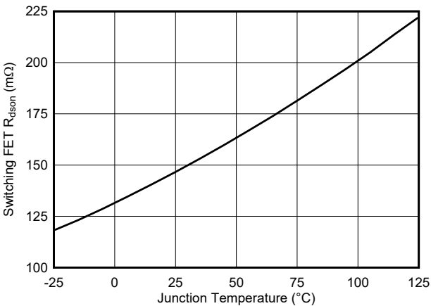
图 6-4. 开关 FET R_{ds(on)} 与结温间的关系
