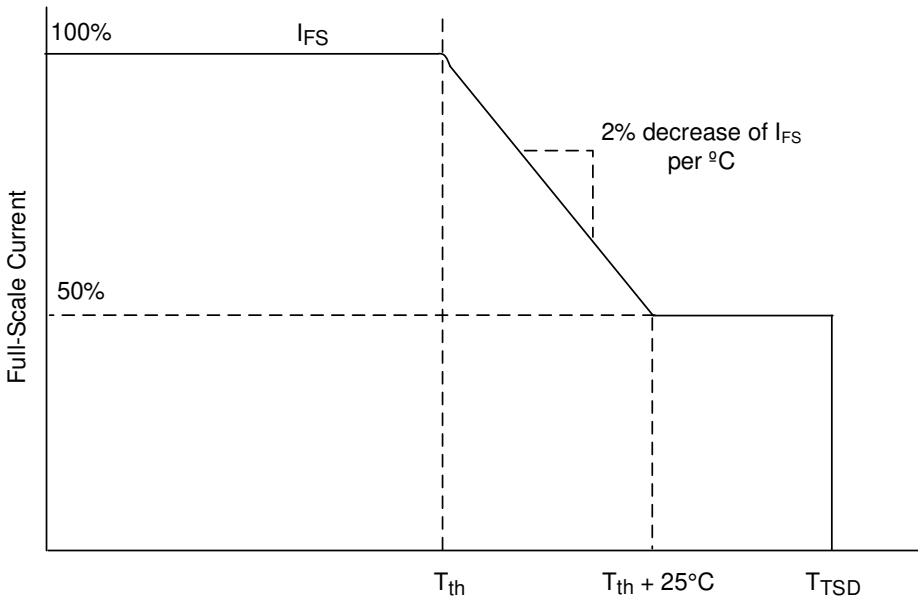
图 7-4. 热折返
