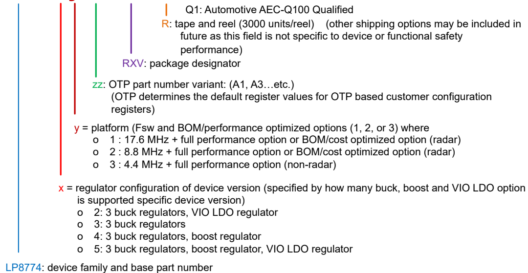
图 4-1. LP8774x-Q1 可订购器件型号方案
