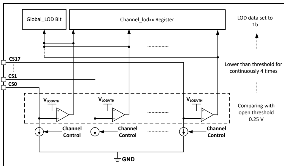
图 8-8. LOD 电路
