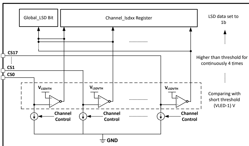
图 8-9. LSD 电路
