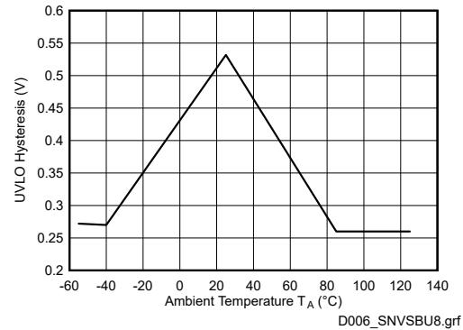
图 7-4. V_{CC} UVLO 迟滞
