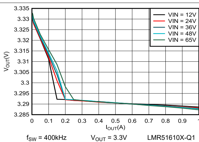
图 6-8. 3.3V Load Regulation
