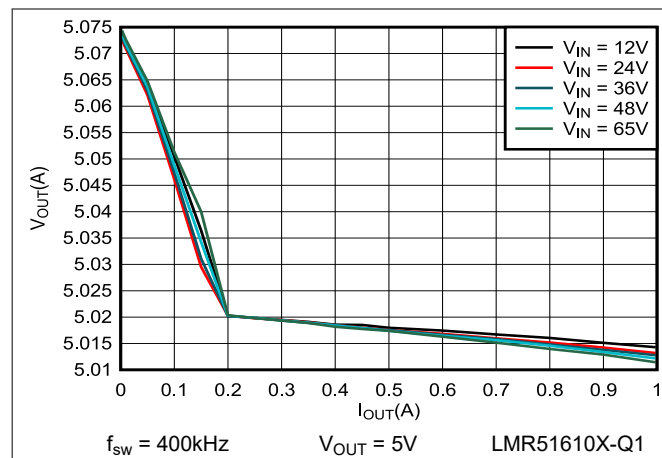
图 6-7. 5V load Regulation
