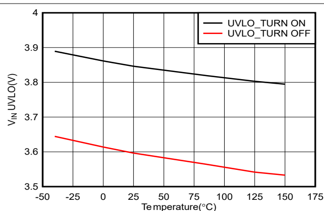
图 6-10. V_{IN} UVLO Versus Temperature
