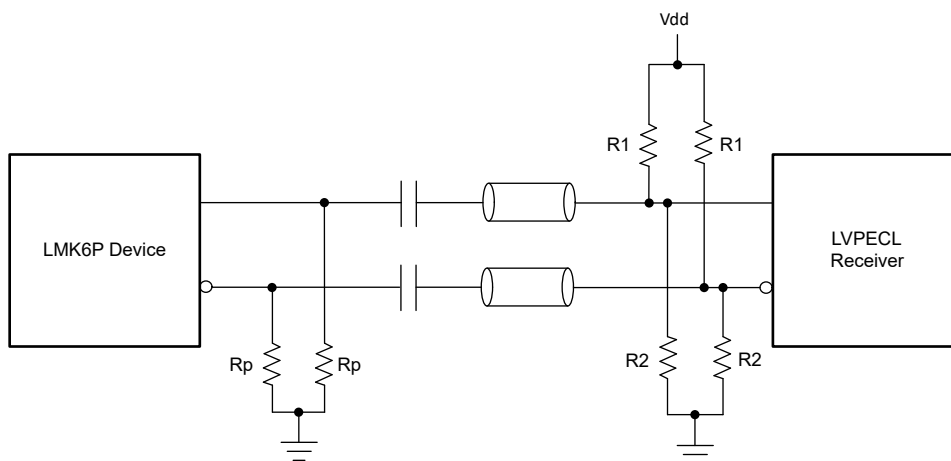
图 8-6. LMK6P 输出交流耦合至带外部端接/偏置的 LVPECL 接收器 (T 型网络)
