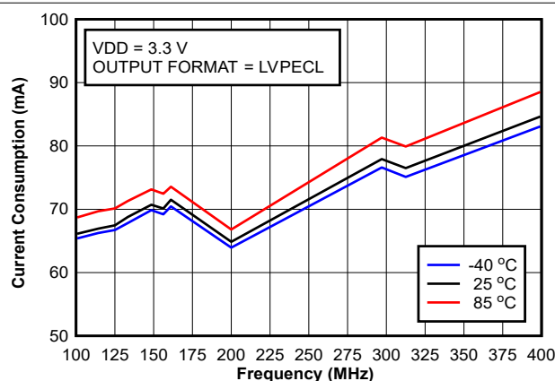
图 6-11. 电流消耗与频率间的关系 (LVPECL、3.3V)
