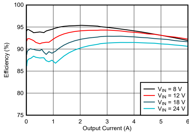
图 8-3. LM634x0-Q1 Efficiency
