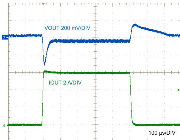
图 8-8. LM634x0-Q1 Load Transient, I_{OUT} = 0A to 6A
