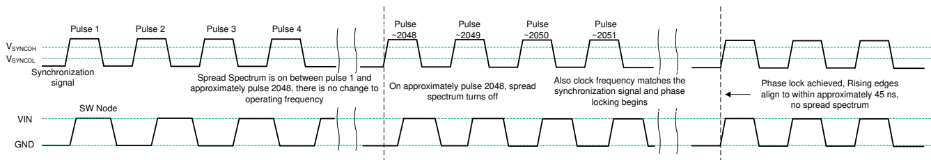
图 7-3. Synchronization Process
