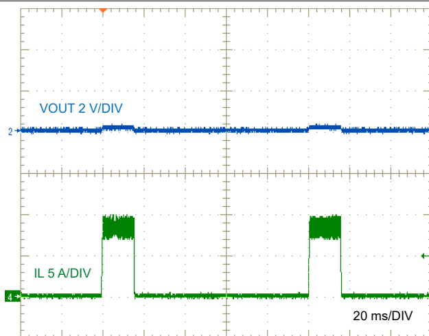
图 8-28. LM634x0-Q1 Short-Circuit Hiccup
