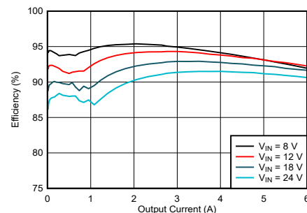
效率， V_{OUT} = 5V ， f_{sw} = 2.1MHz ，LM63460-Q1
