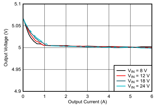
图 8-4. LM634x0-Q1 Load and Line Regulation
