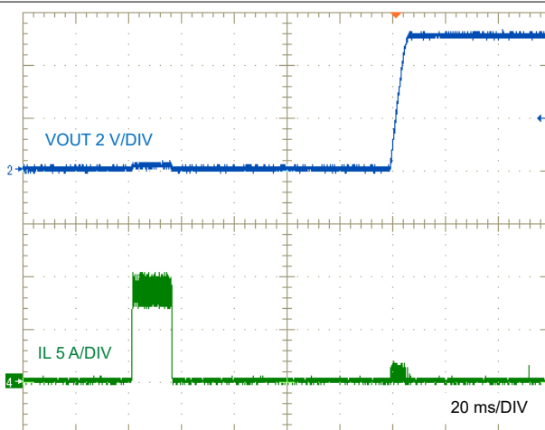
图 8-10. LM634x0-Q1 Short-Circuit Recovery to No Load
