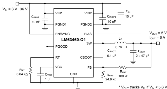
典型电路原理图
