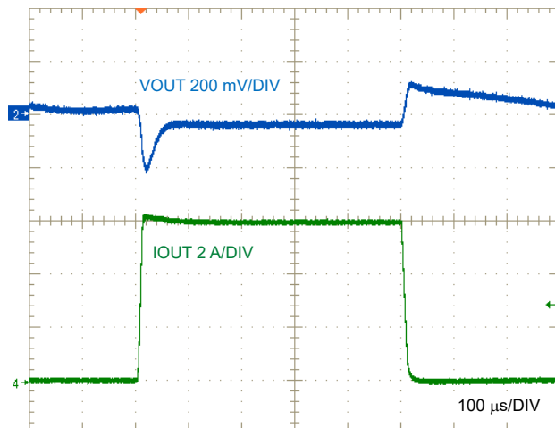
图 8-27. LM634x0-Q1 Load Transient, I_{OUT} = 0A to 6A
