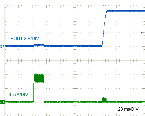
图 7-11. Short-Circuit Recovery
