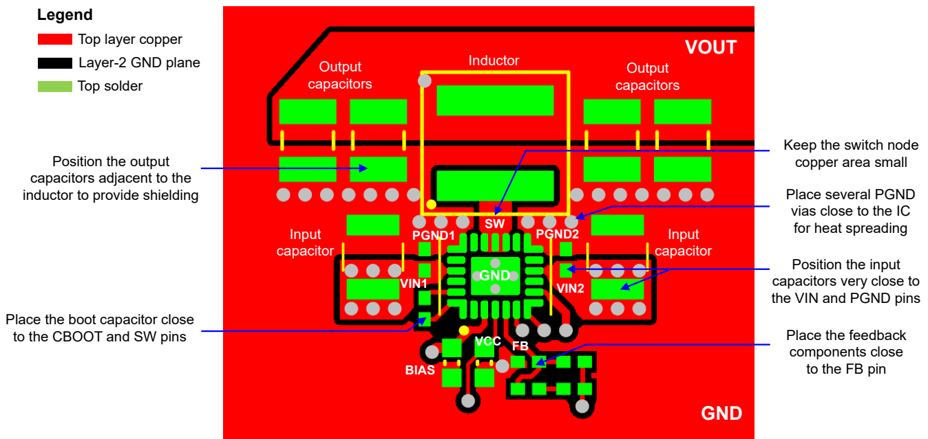
图 8-31. PCB Layout Example
