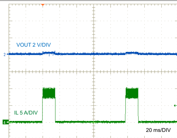
图 8-9. LM634x0-Q1 Short-Circuit Hiccup
