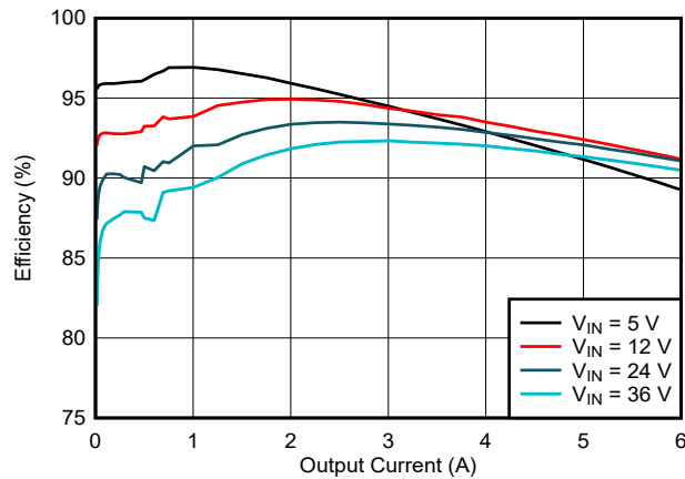
图 8-22. LM634x0-Q1 Efficiency
