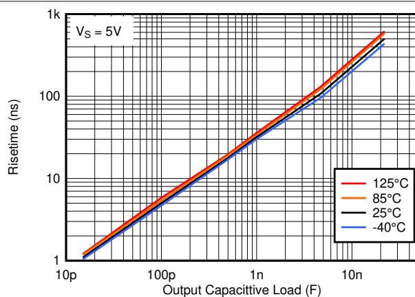
图 6-11. Rise time vs. Capacitive Load
