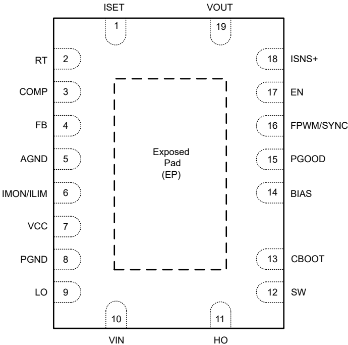
图 4-1. 19 引脚 VQFN RGY 封装（顶视图）
