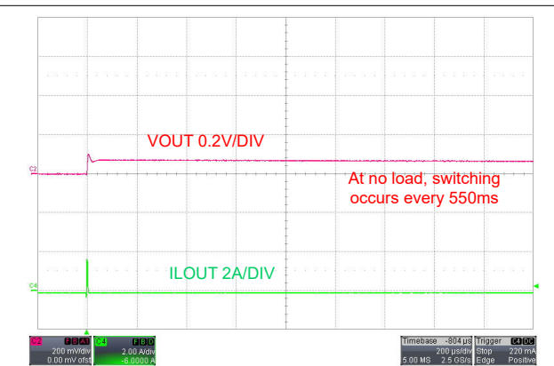
图 7-10. PFM 模式下的空载运行， V_{SUPPLY} = 12V
