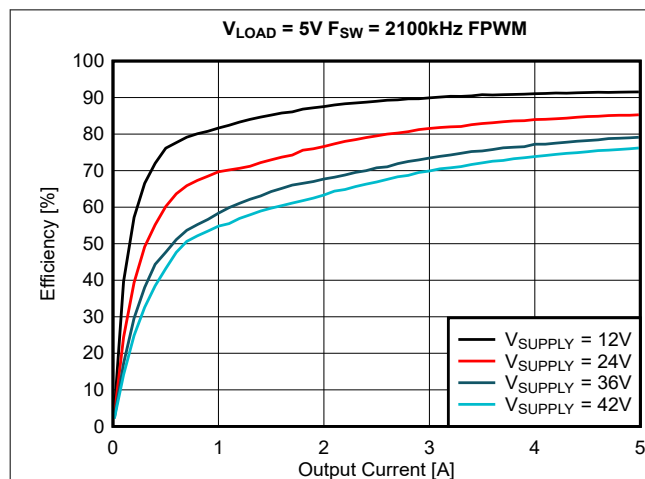
图 7-5. FPWM 模式效率，线性标度
