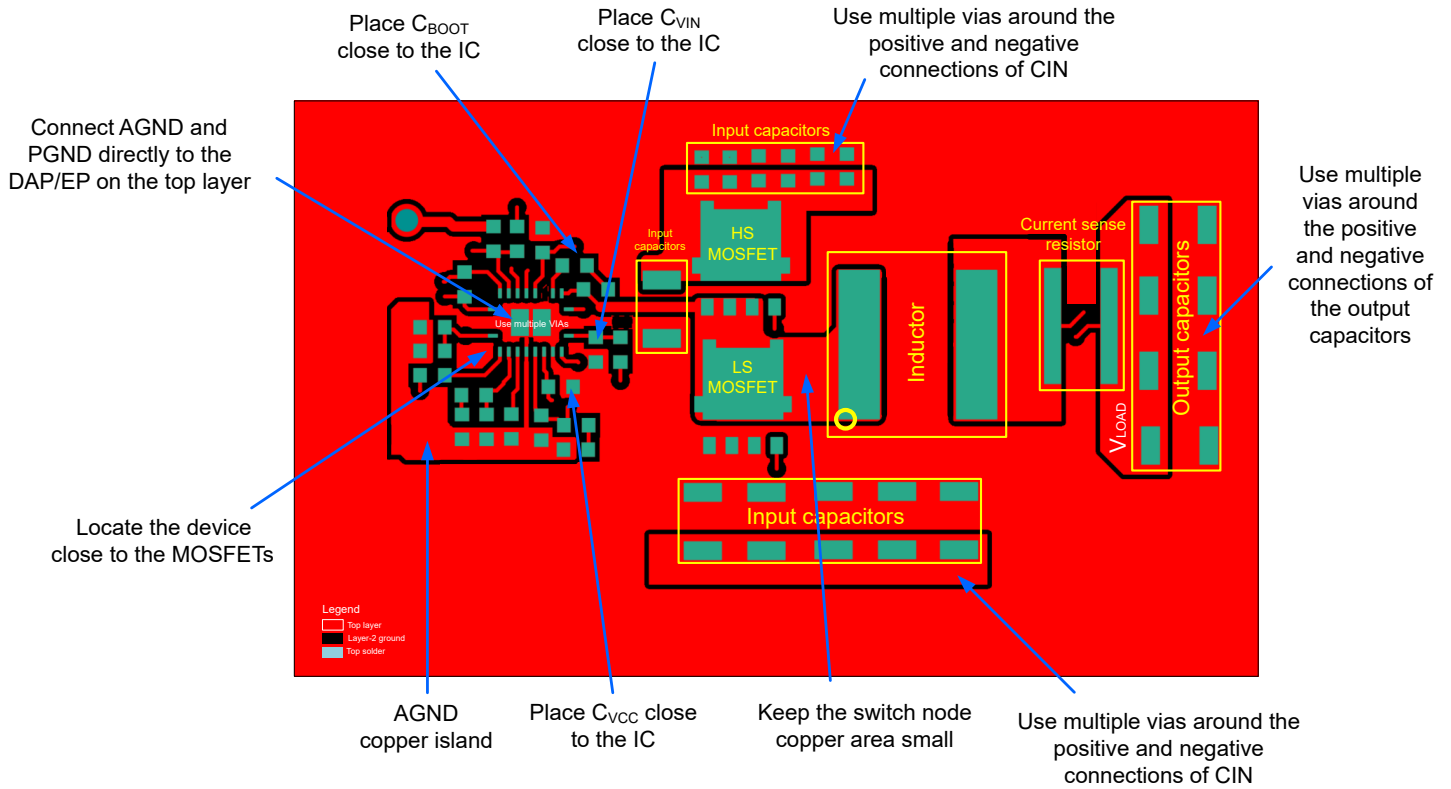
图 7-16. PCB 顶层
