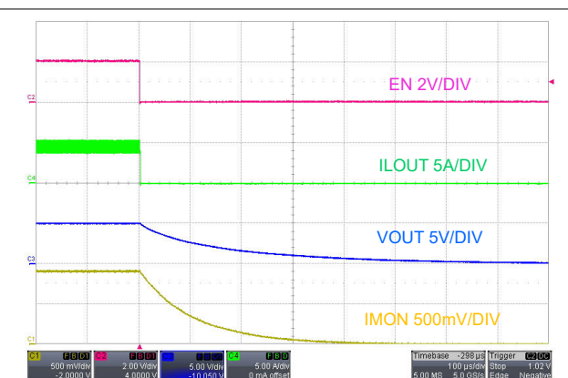
图 7-8. 关断，EN 关闭， V_{SUPPLY} = 12V ， I_{LOAD} = 5A 电阻负载
