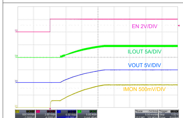
图 7-7. 启动，EN 开启， V_{SUPPLY} = 12V ， I_{LOAD} = 5A 电阻负载
