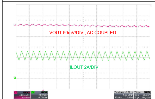
图 7-9. 输出纹波， V_{SUPPLY} = 12V
